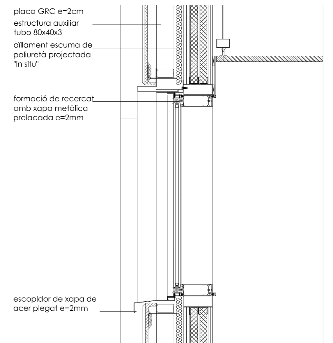
DET.B. e 1:5
