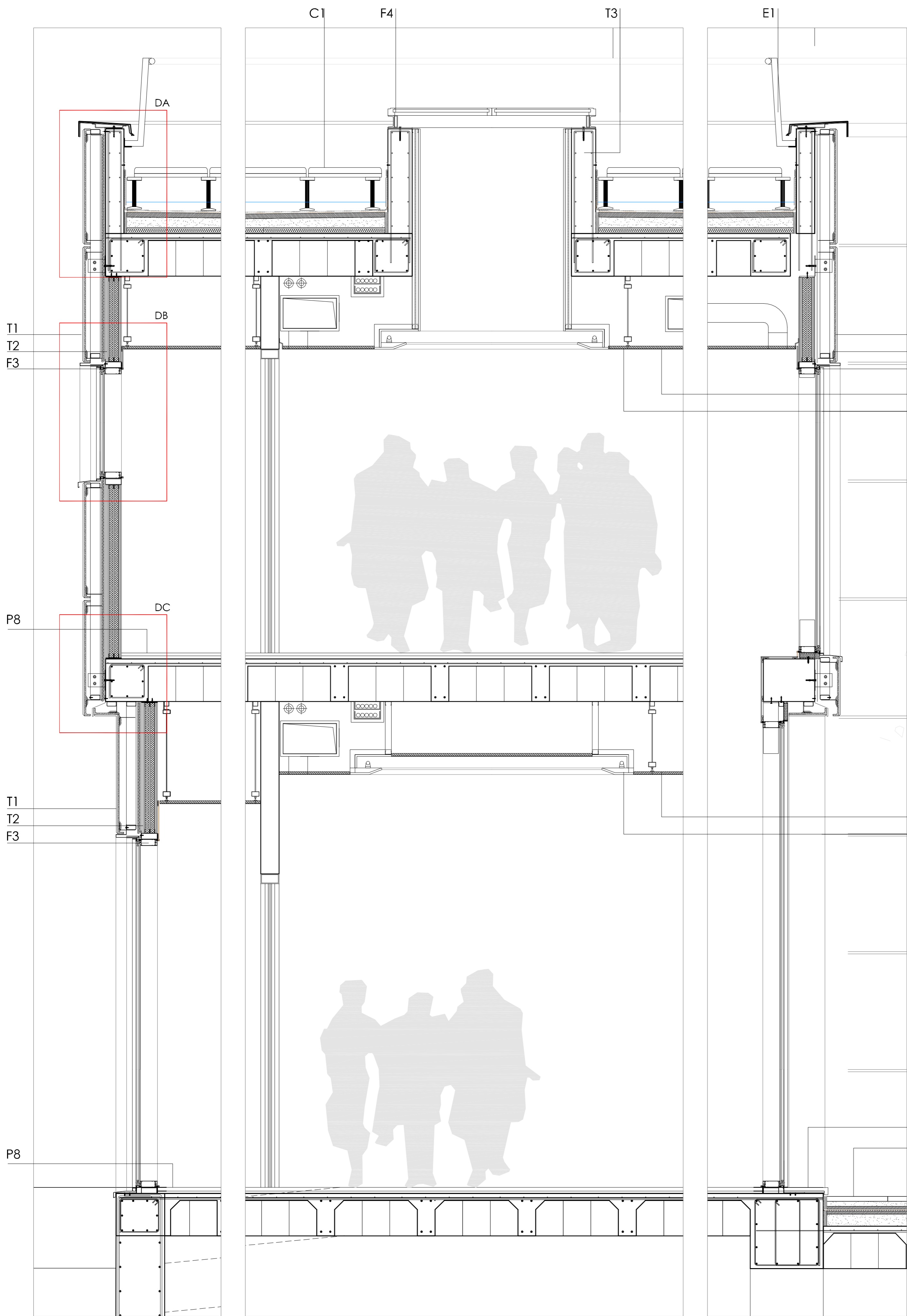
DET.1. e 1:20
