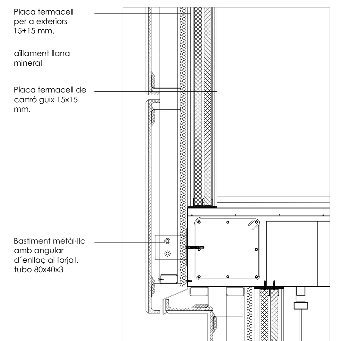
DET.C. e 1:5
