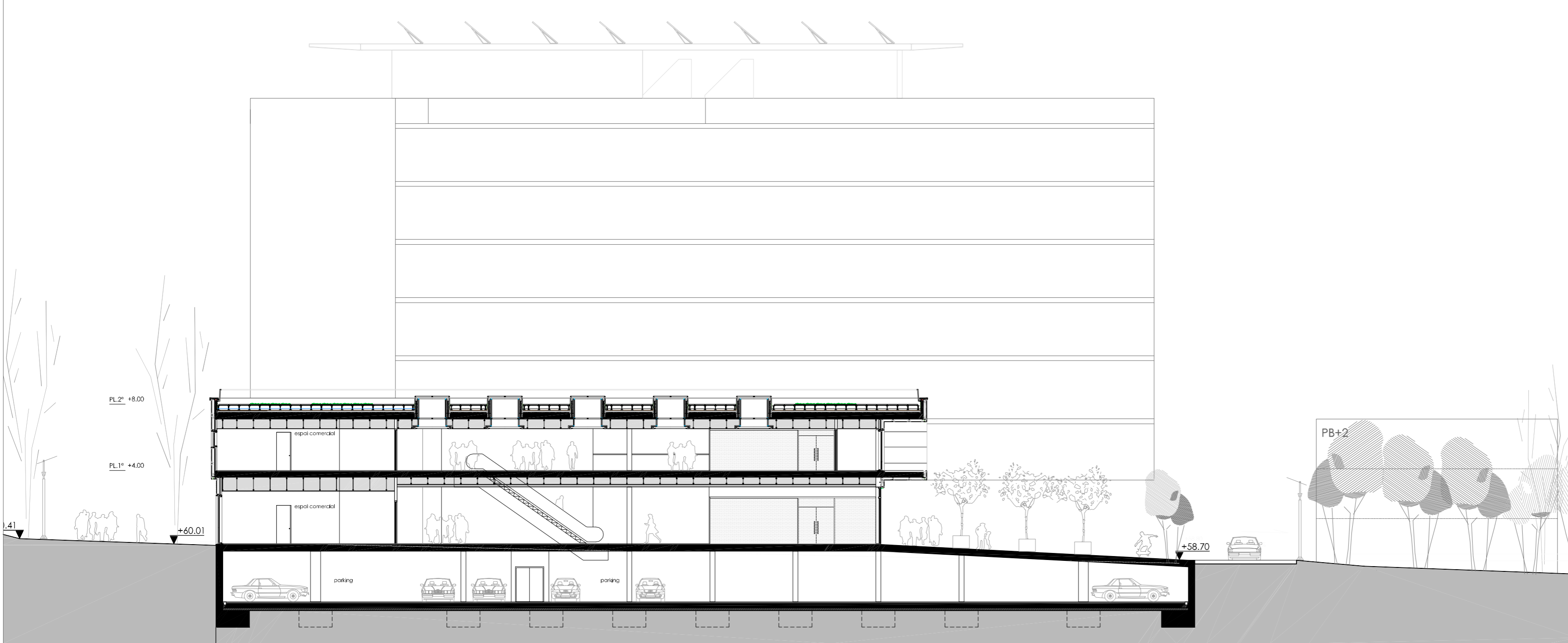
SECCIÓ CC. e 1:200
