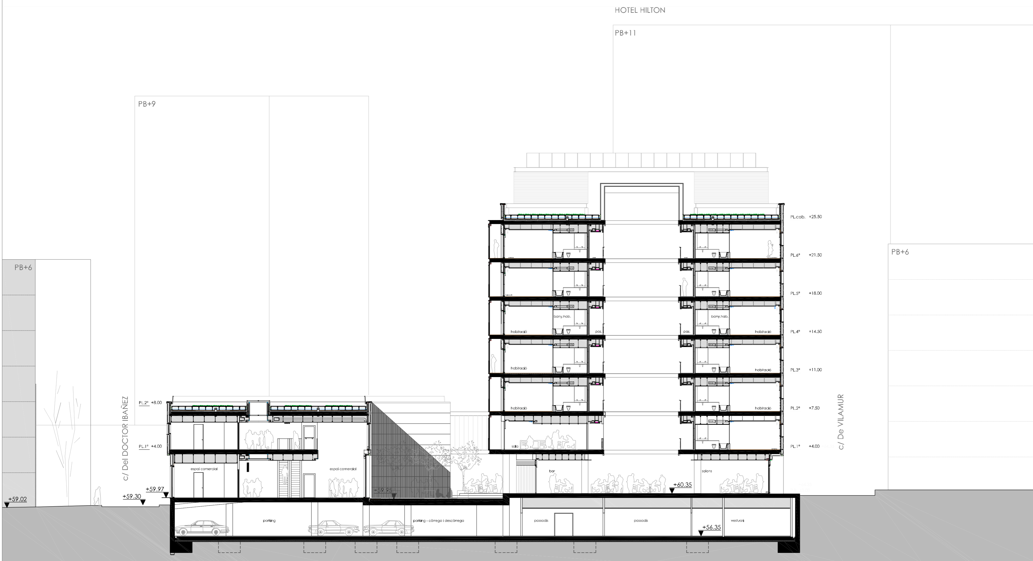
SECCIÓ BB. e 1:200
