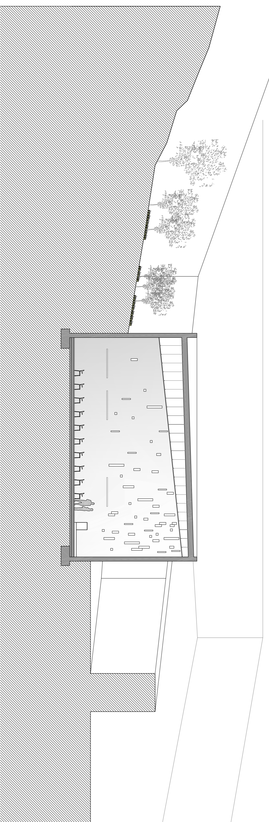
_secció FF'
