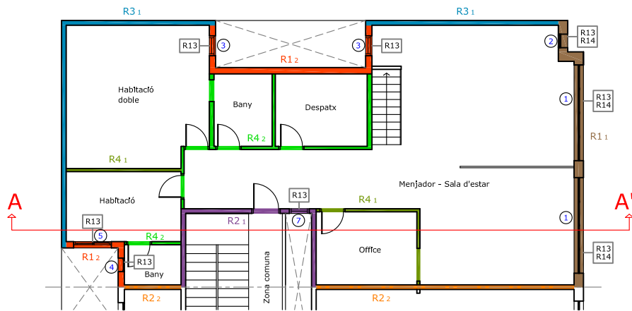
PLANTA PRIMERA
