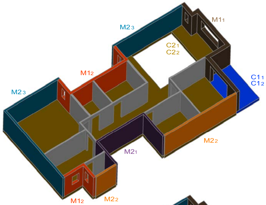
PLANTA SEGONA
