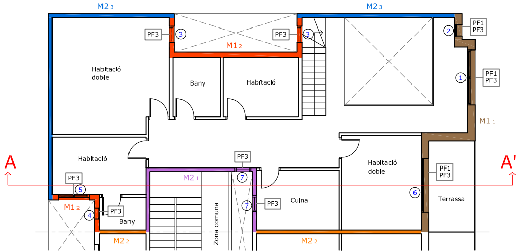
PLANTA SEGONA
