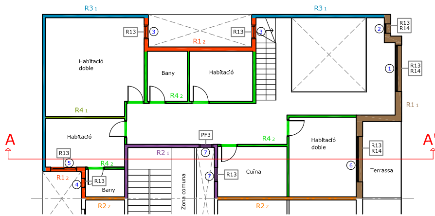
PLANTA SEGONA
