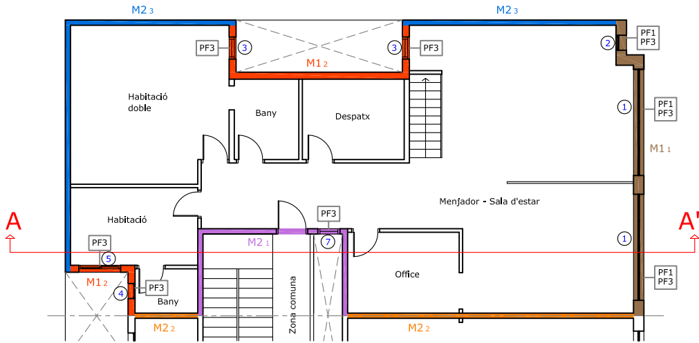
PLANTA SEGONA
