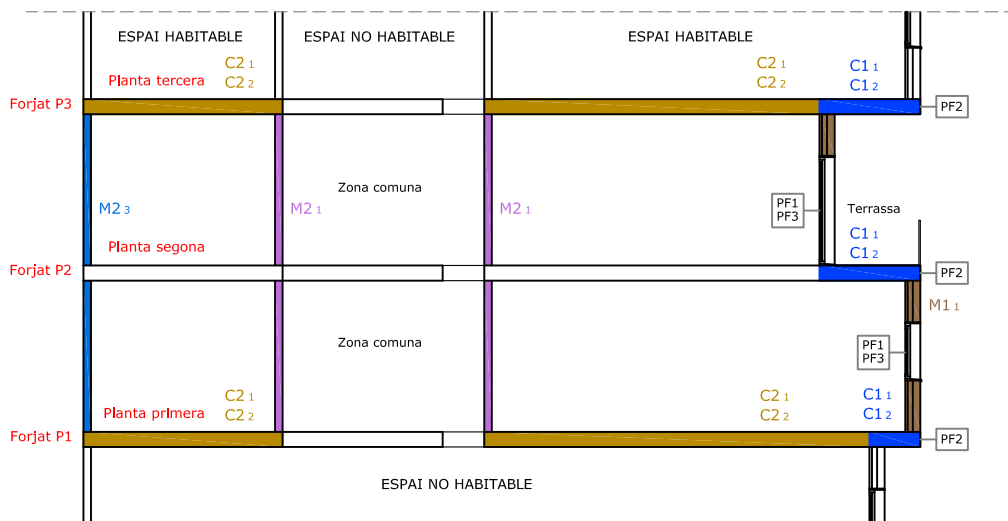
SECCIÓ A-A'
