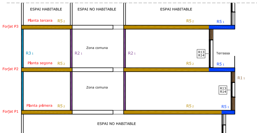
SECCIÓ A-A'
