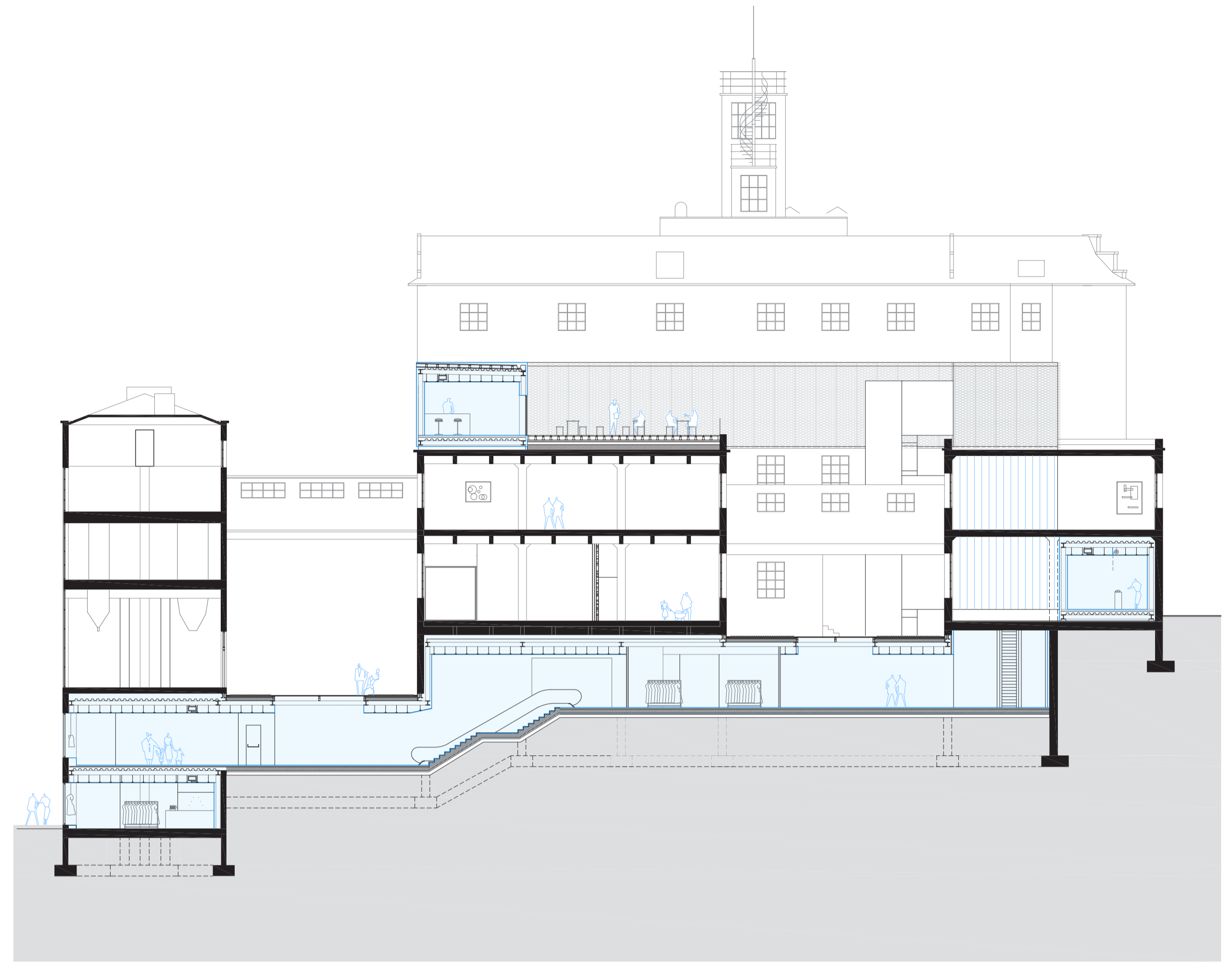
sección s3
