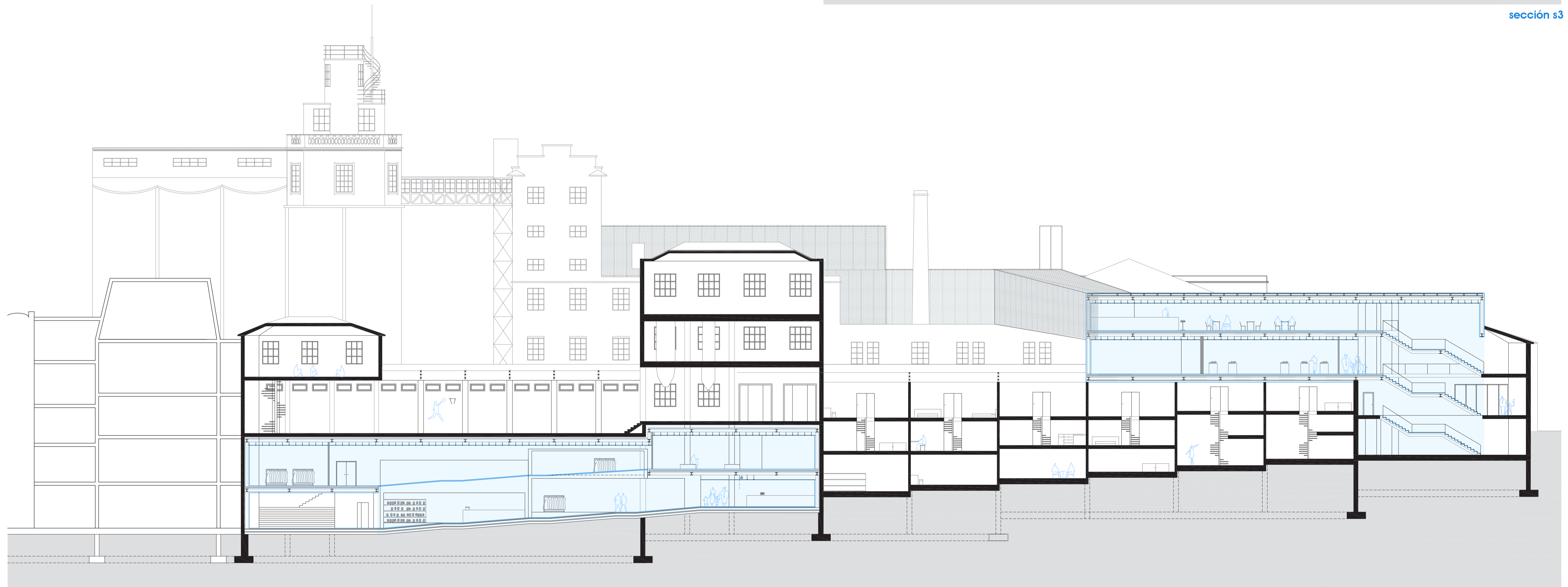
sección s4
