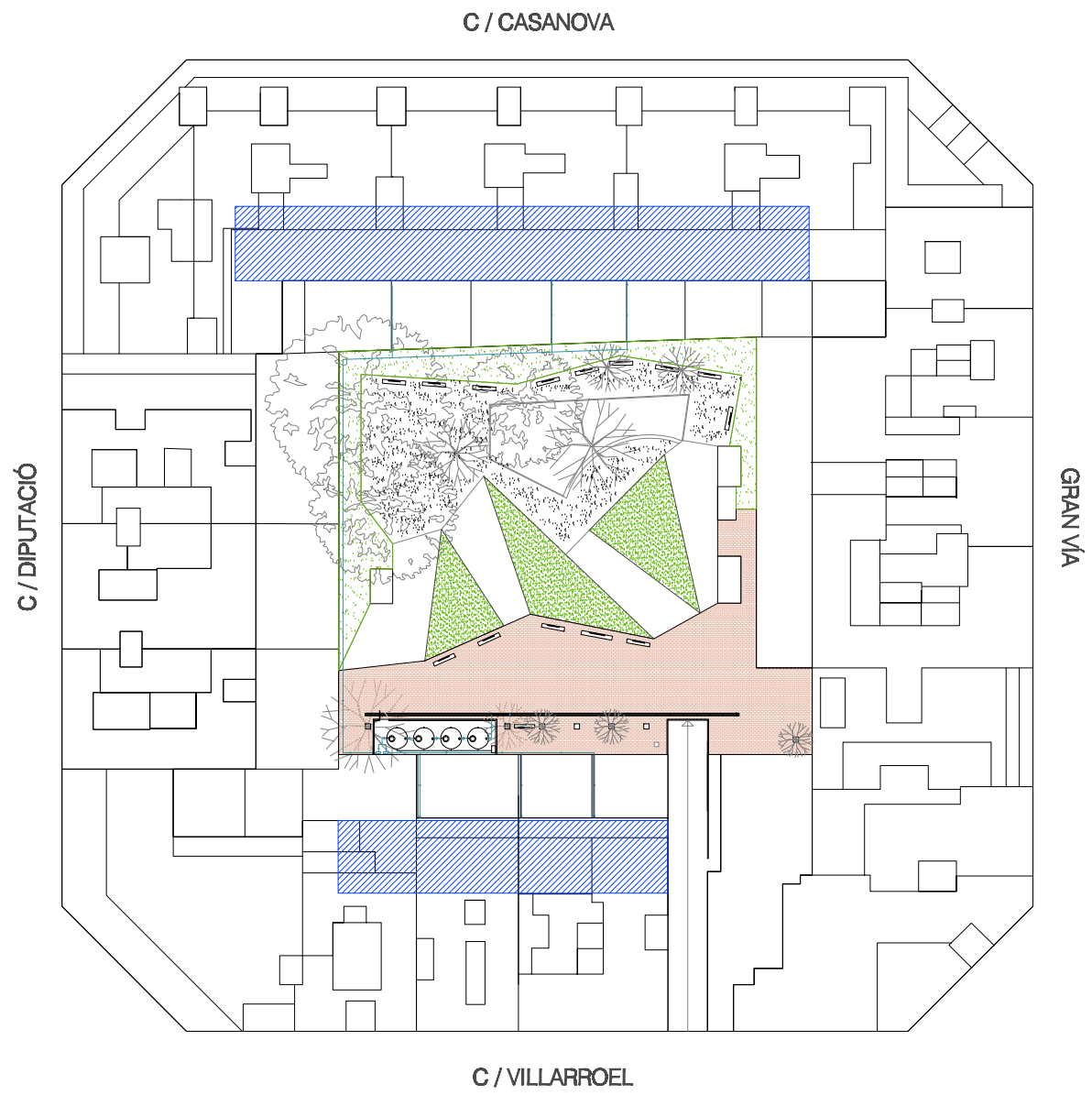
Planta con Sistema de Recogida de Aguas Pluviales y superficie de cubiertas de captación.
