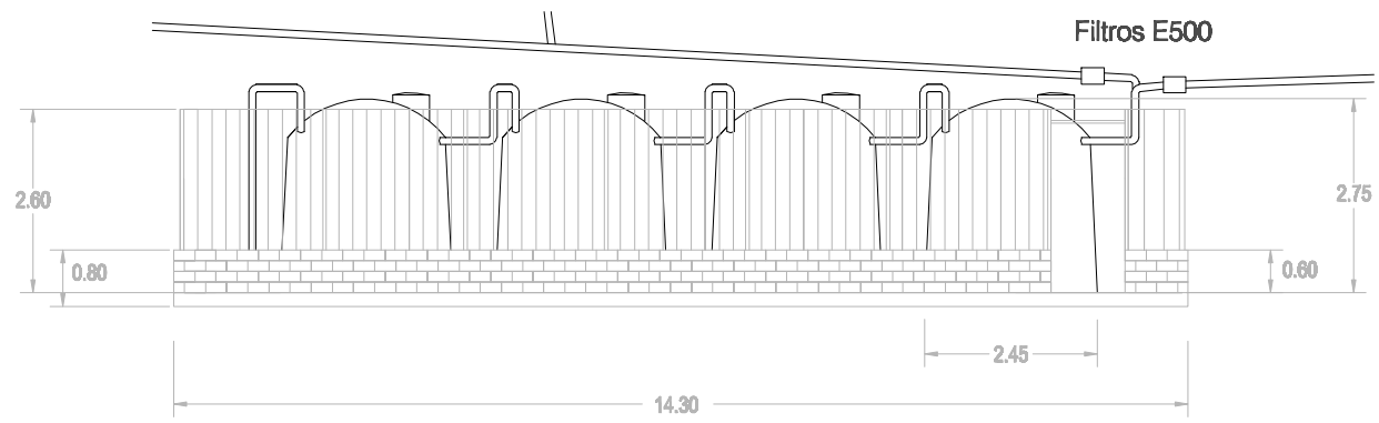
Alzado frontal de depósitos y vallado
