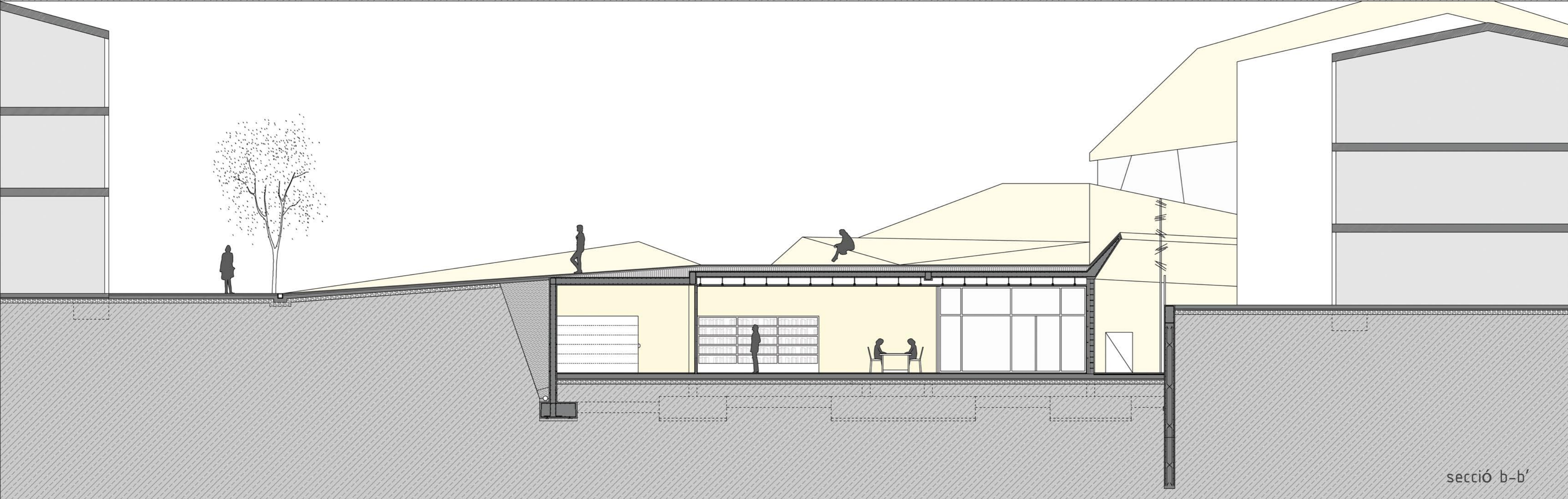
secció a-a'
