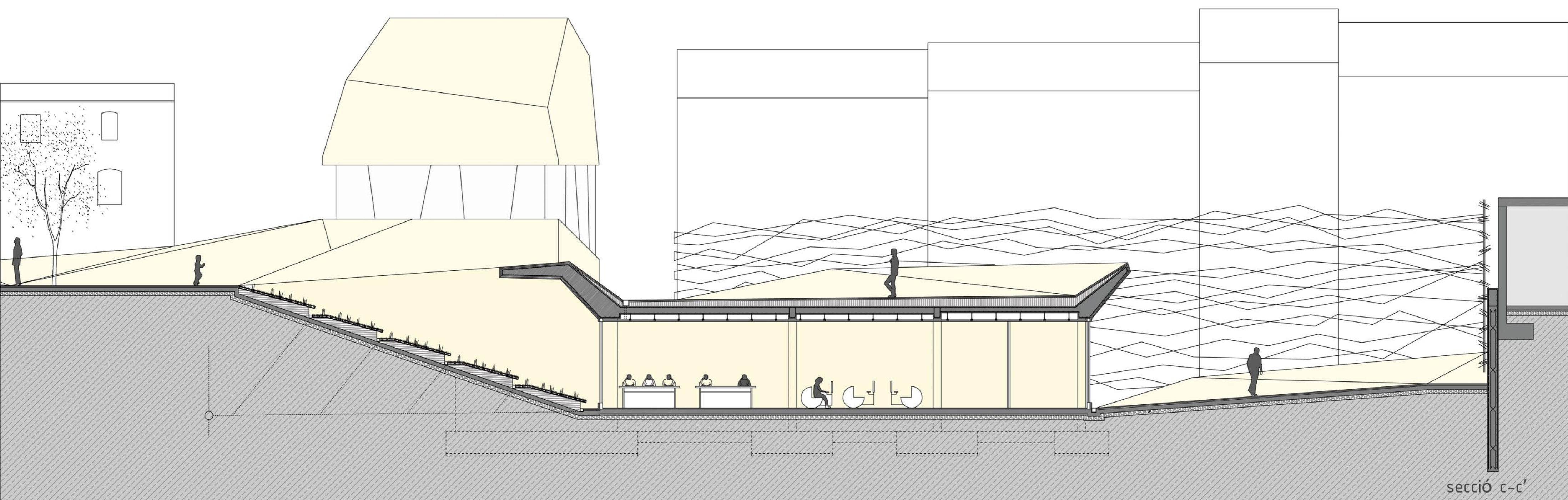
secció b-b'
