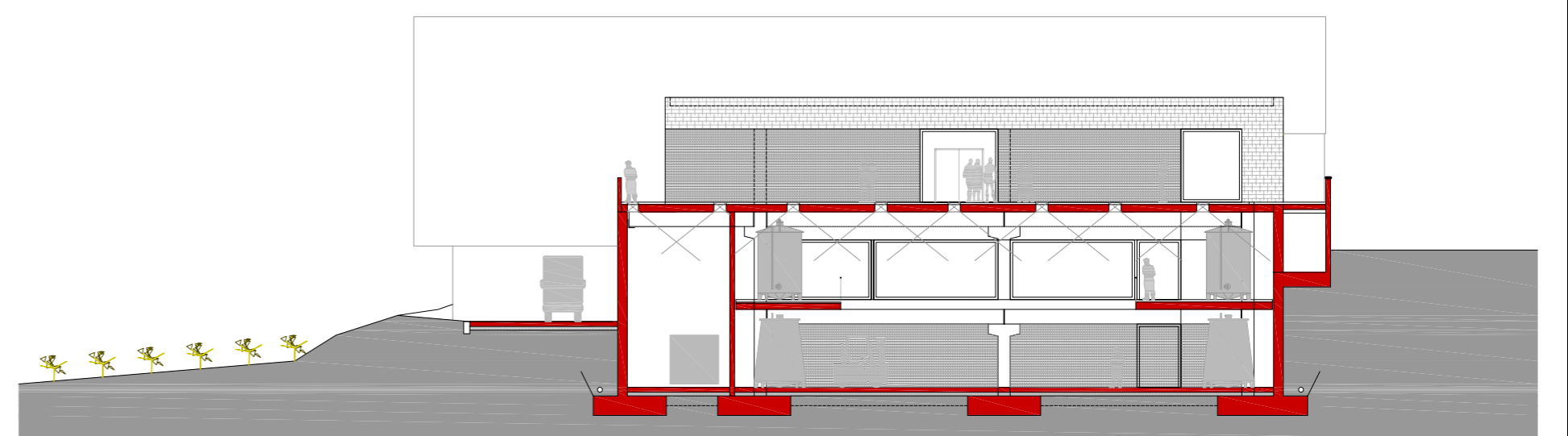
SECCIÓ E
