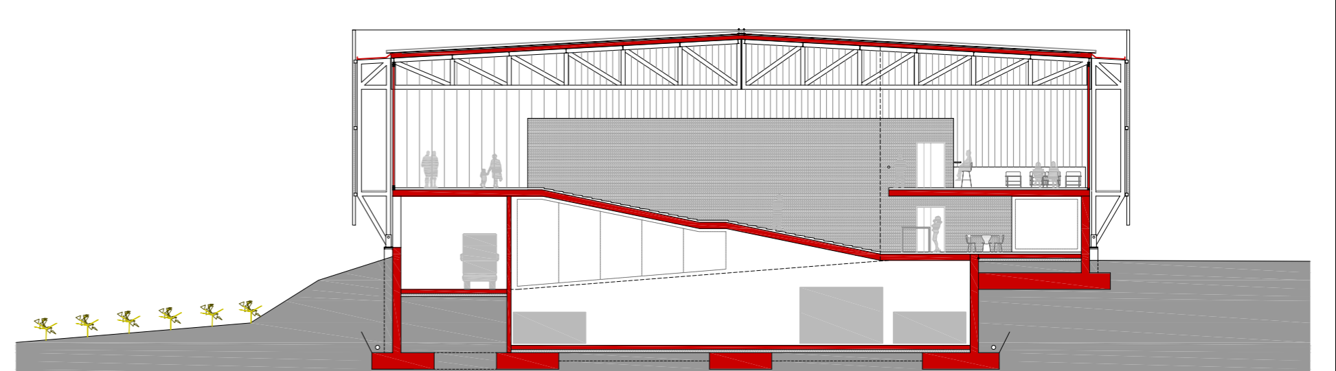
SECCIÓ A
