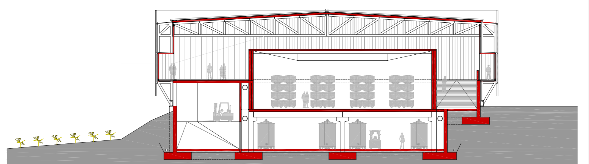
SECCIÓ C
