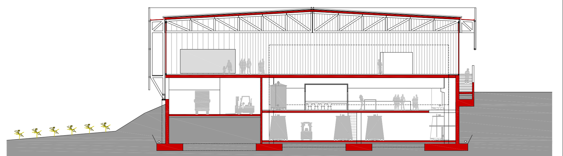
SECCIÓ D
