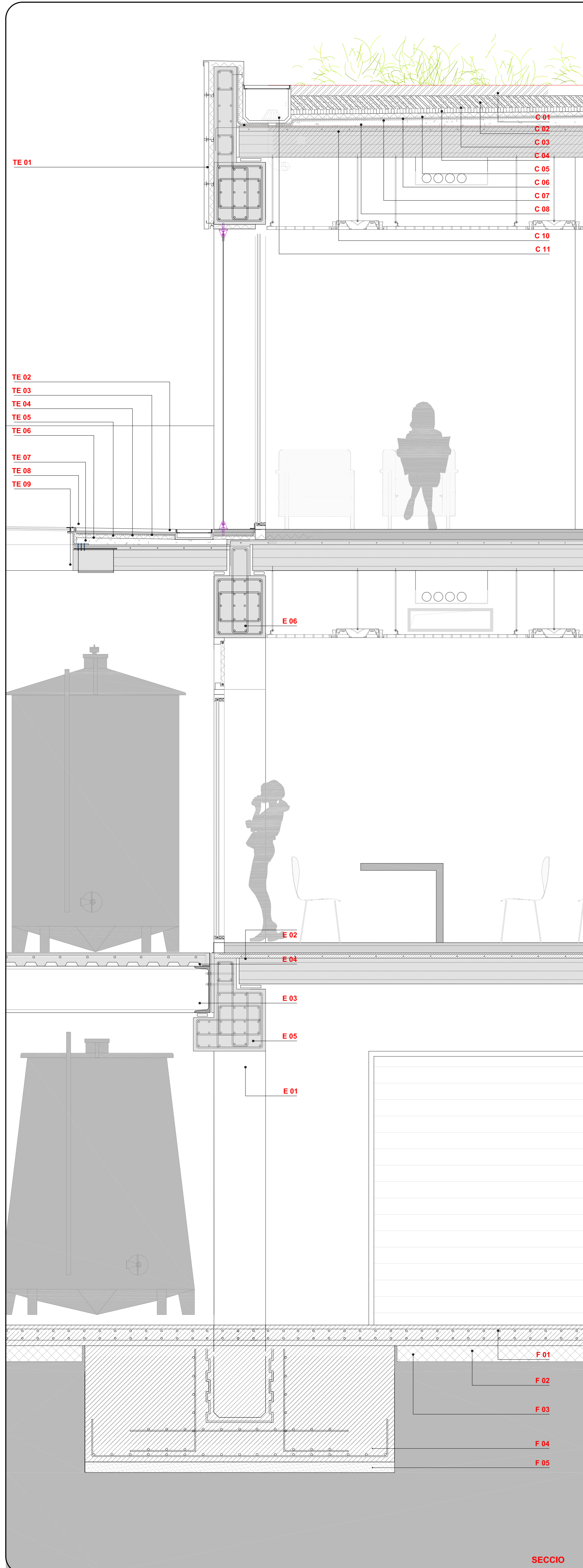
SECCIÓ
