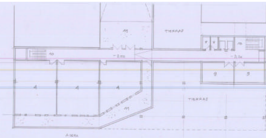
PLANTA SEMISOTANO -1 1/200
