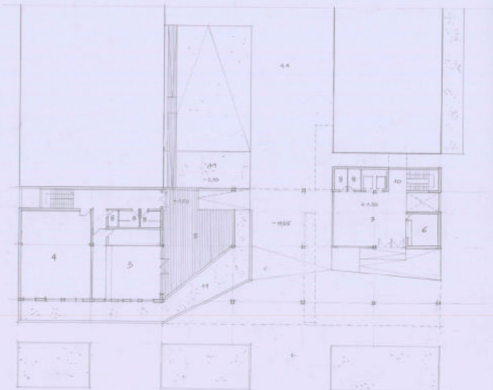
PLANTA SEMISOTANO -1 1/200
