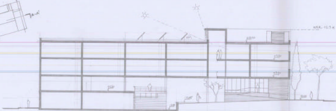
SECCIÓN 1-1' 1/100
