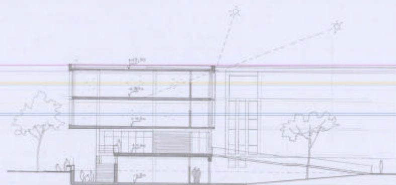
SECCIÓN A-A 1/100
