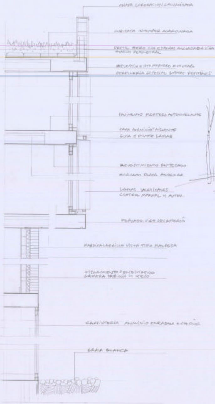
DETALLE CONSTRUCTIVO - 1/20
