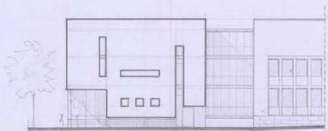
ALZADO C/ TPU ESC. 1/250
