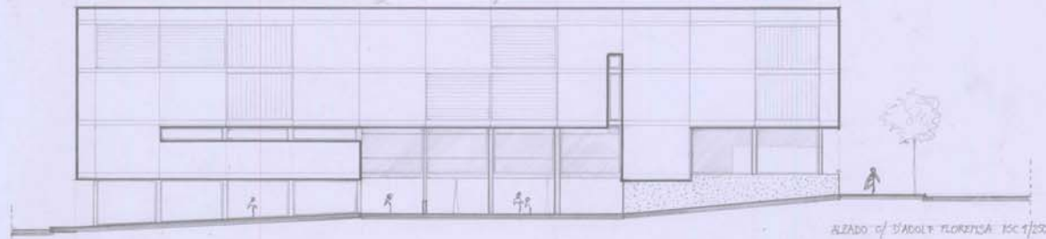
ALZADO C/ DAROLT FLORENSA ESC. 1/250
