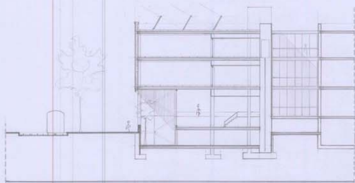
SECCION A-A ESC. 1/250
