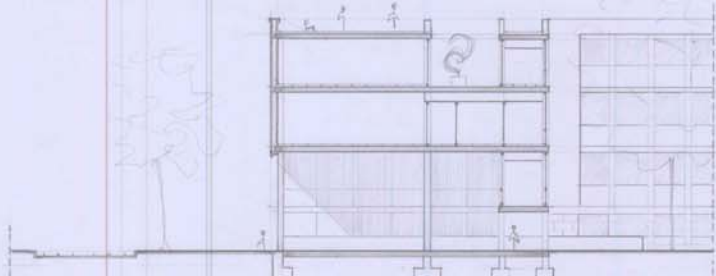
SECCION A-A ESC. 1/250
