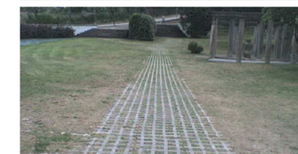
Imatges on es pot apreciar el tipus de paviment permeable emprat en la proposta, són peces prefabricades de formigó.
