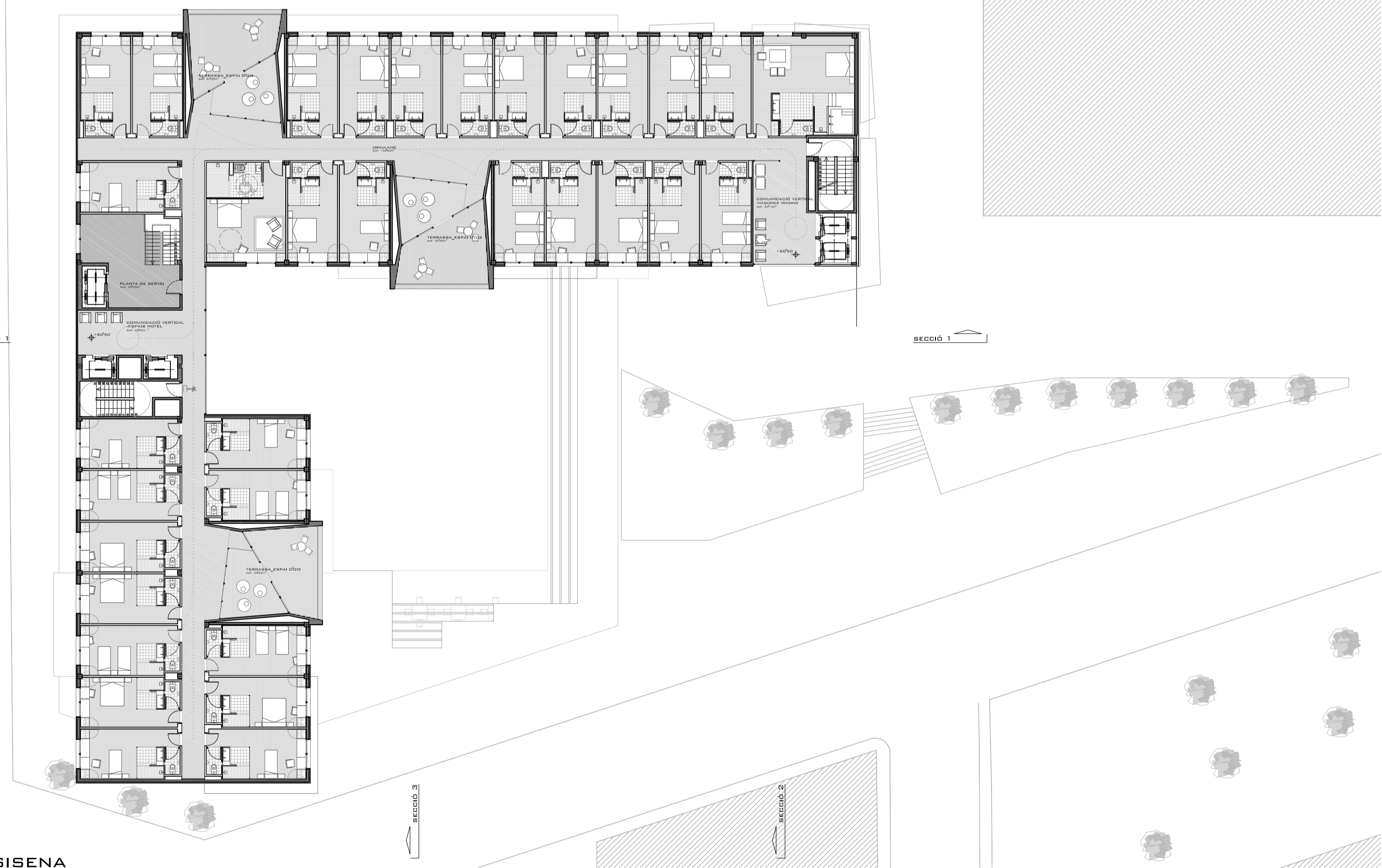
PLANTA SISENA
