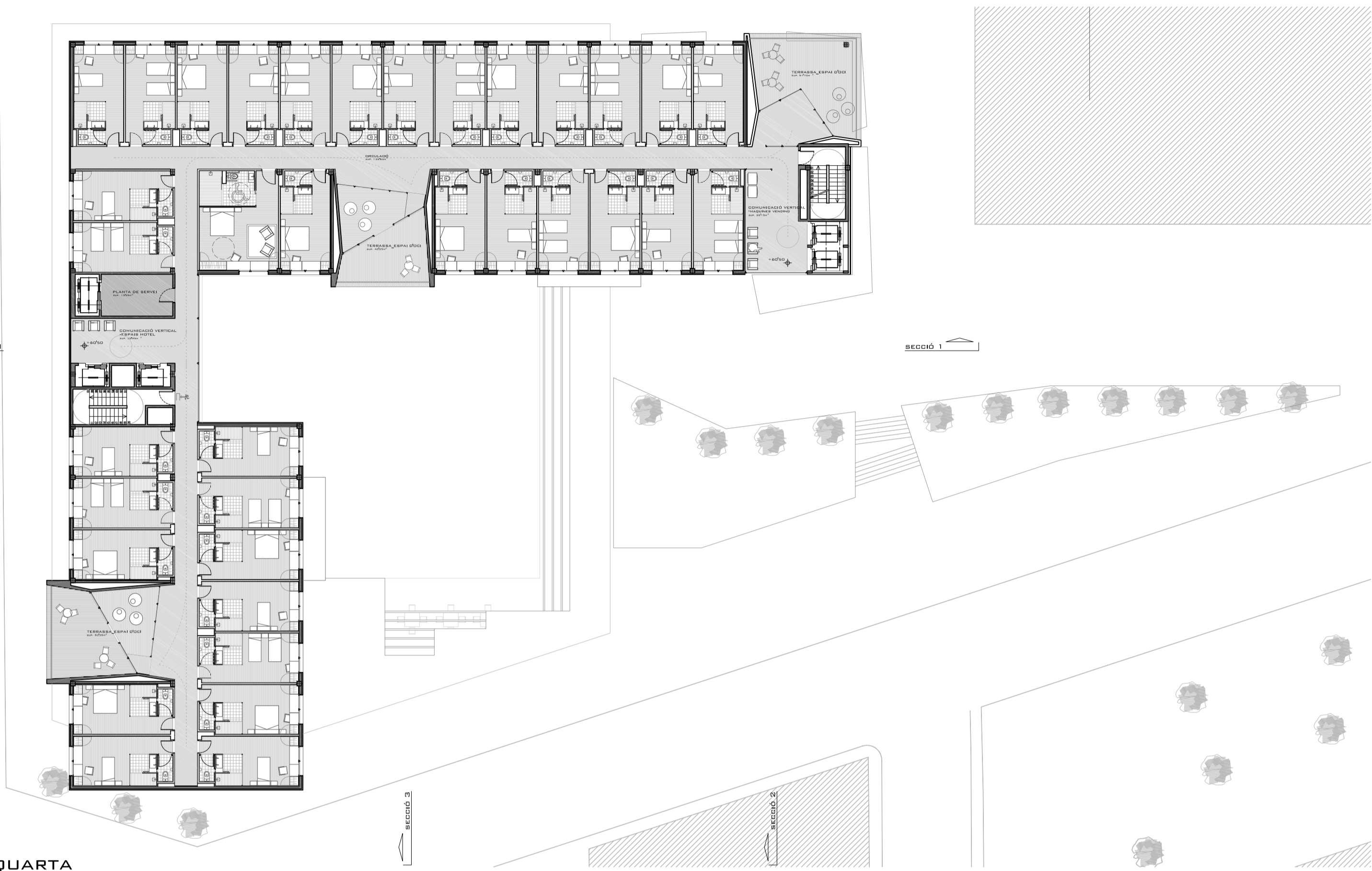
PLANTA QUARTA
