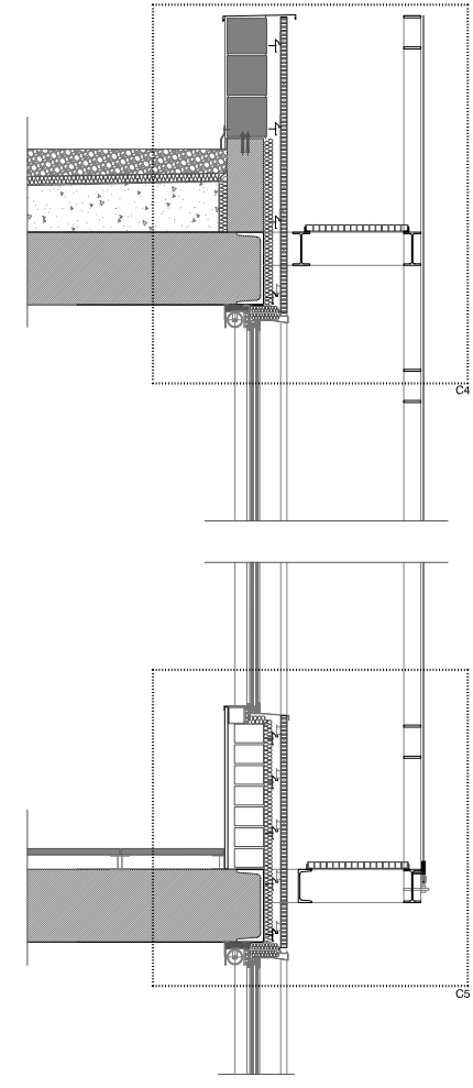
malla metàl·lica e 1/20
