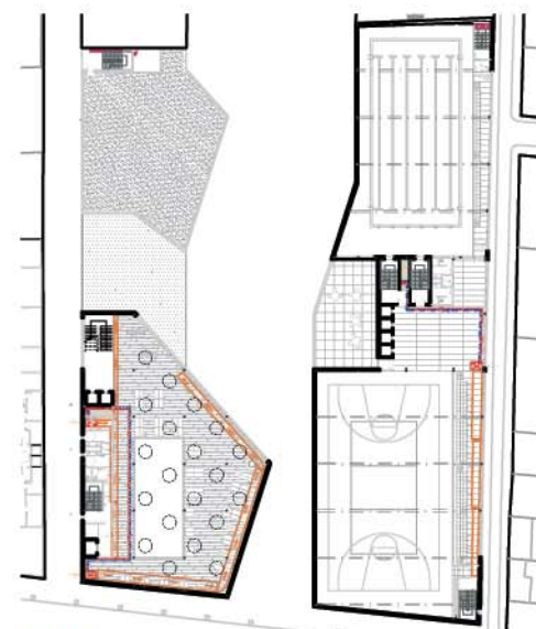
PLANTA 04 e : 1/500
