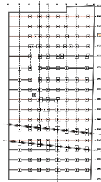
PLANTA FONAMENTS Nivell -6.00m
