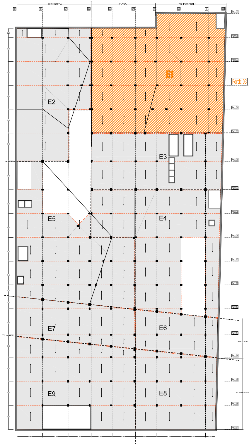
SOSTRE PLANTA SOTERRANI -1 Nivell ±0.00m e. 1/200
