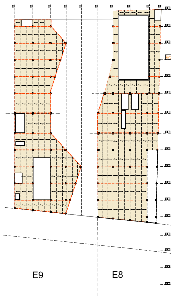
SOSTRE PLANTA SEGONA Nivell +10.80m
