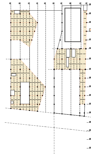
SOSTRE PLANTA TERCERA Nivell +14.40m
