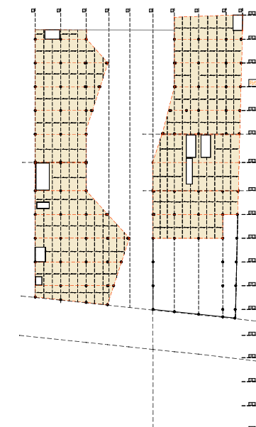
SOSTRE PLANTA PRIMERA Nivell +7.20m
