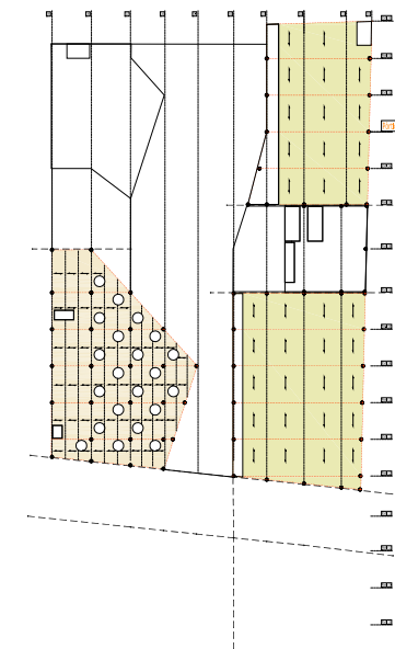
SOSTRE PLANTA QUARTA Nivell +18.80m
