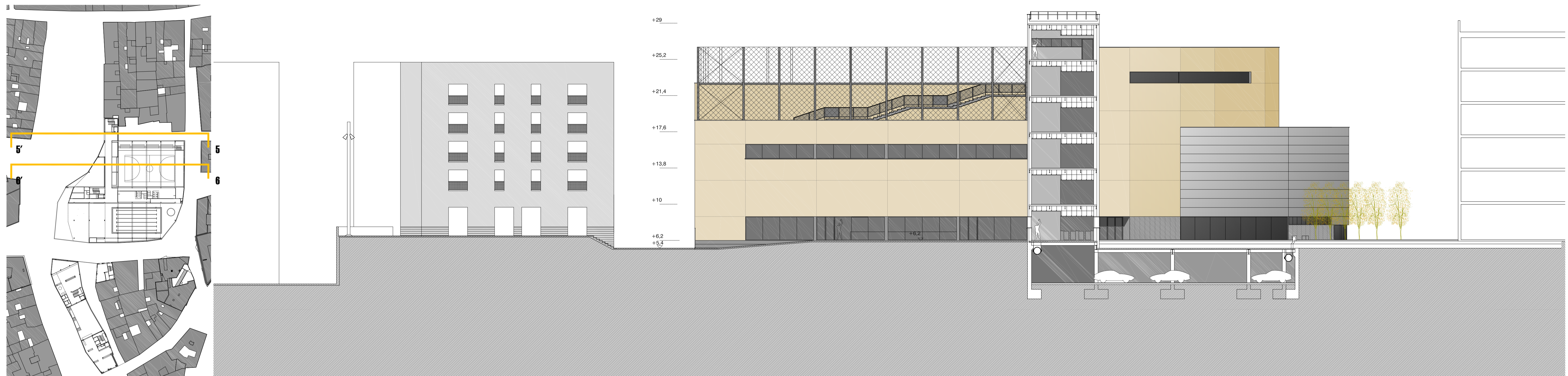
SECCIÓN 5-5'. 1:200.
