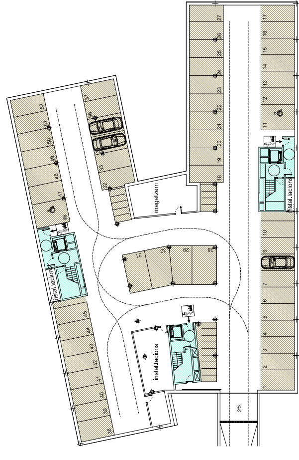
PLANTA APARCAMENT
