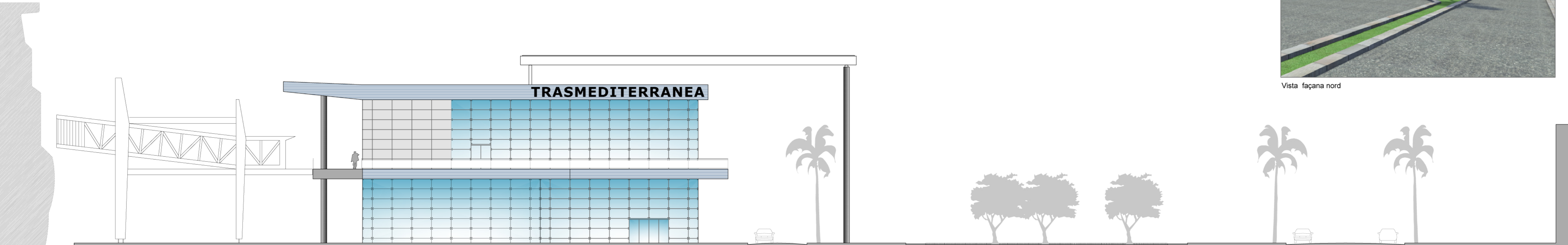
FAÇANA NORD E:1/200
