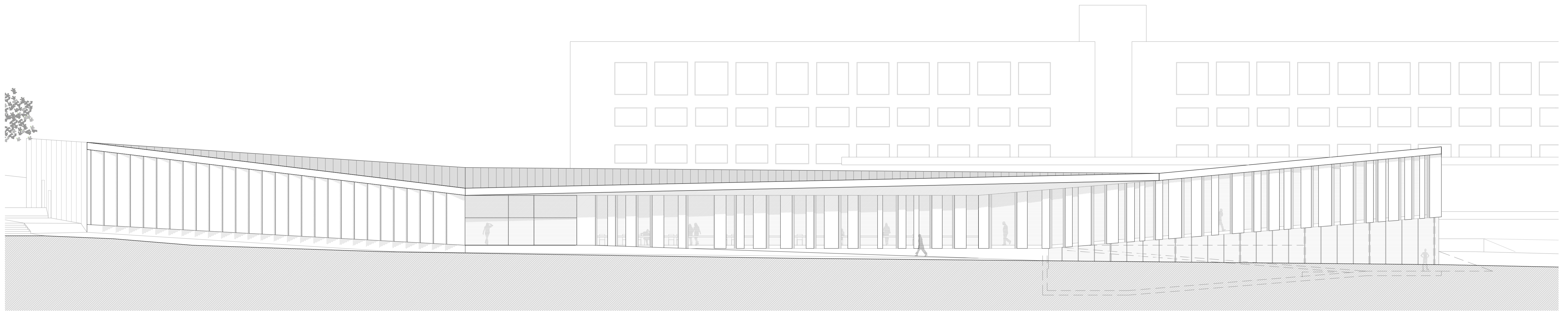
ALÇAT 1 - ALÇAT SUD - FAÇANA DEL FOYER, OPACA DES DE TOTS ELS PUNTS DE VISTA EXCEPTE UN; PECES DE GRC PARAL·LELES SUBJECTADES AMB LA SEVA SUBESTRUCTURA A TERRA I BIGA LONGITUDINAL SUPERIOR FAÇANA CIRCULACIÓ, COMBINATÓRIA OPAC/VIDRE AMB PECES 'U' DE GRC. LA PROPORCIÓ OPAC/VIDRE VARIA AMB LES CONDICIONS A QUE S'ENFRONTA LA FAÇANA; MÉS VIDRE SOTA EL PORXO, MENYS AL DESCOBERT FAÇANA PS1, TOTALMENT TRANSPARENT AMB SISTEMA DE MUNTANTS I TRAVESSERS. EL VIDRE ARRIBA A LA LÍNIA DE PAVIMENT EXTERIOR, SEPARAT PER UNA FRANJA DE DESGUÀS
