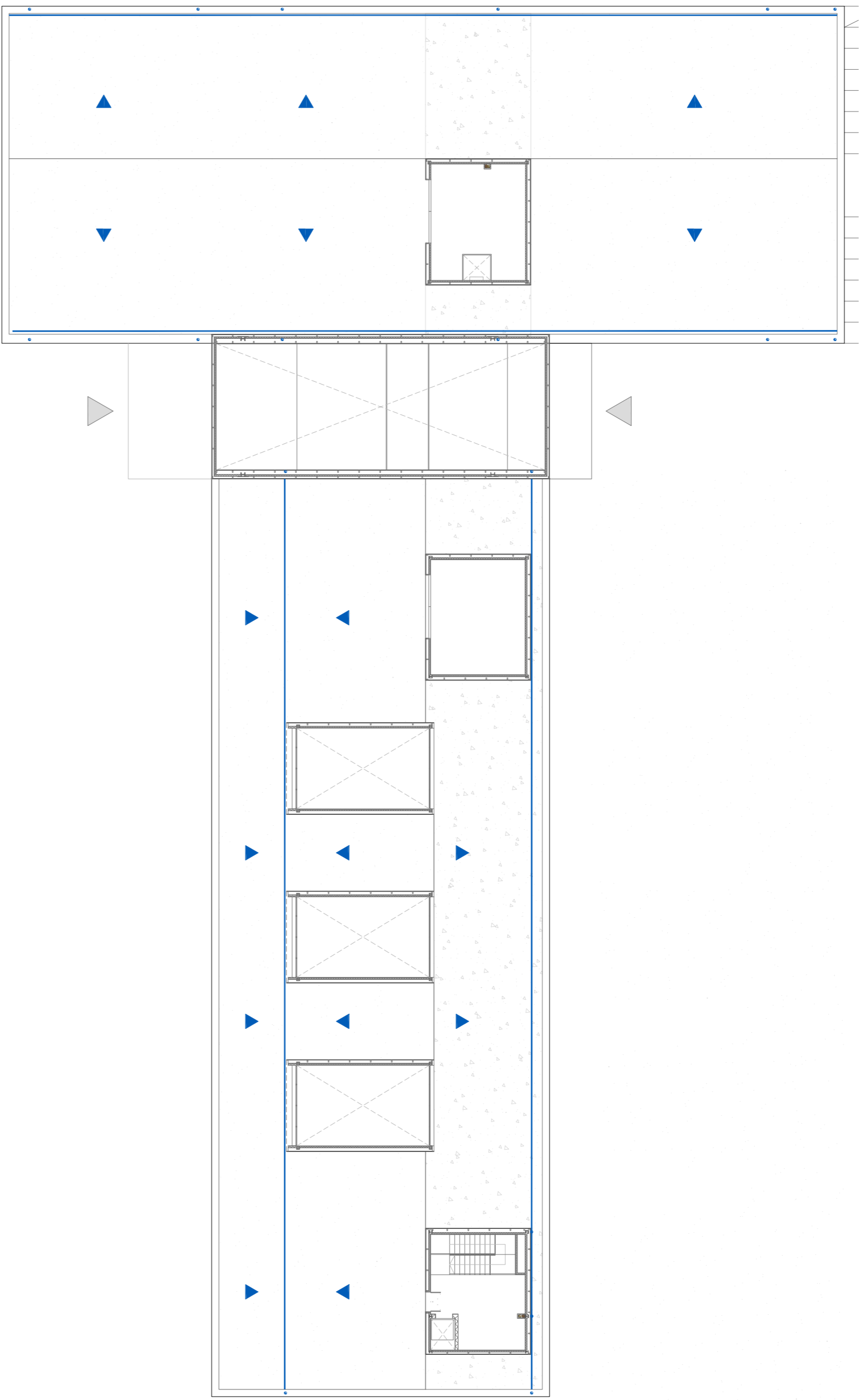
PLANTA COBERTA 1/250
