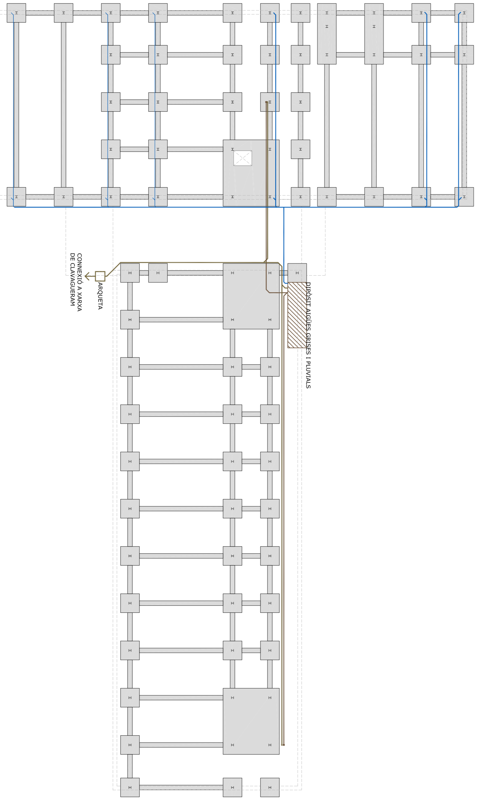
PLANTA FONAMENTS 1/250
