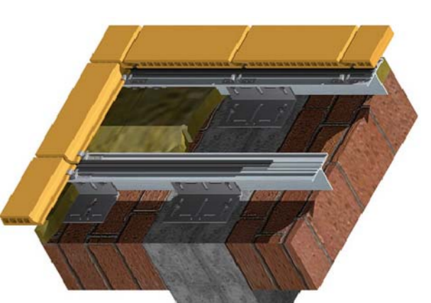
SISTEMA DE FAÇANA VENTILADA
