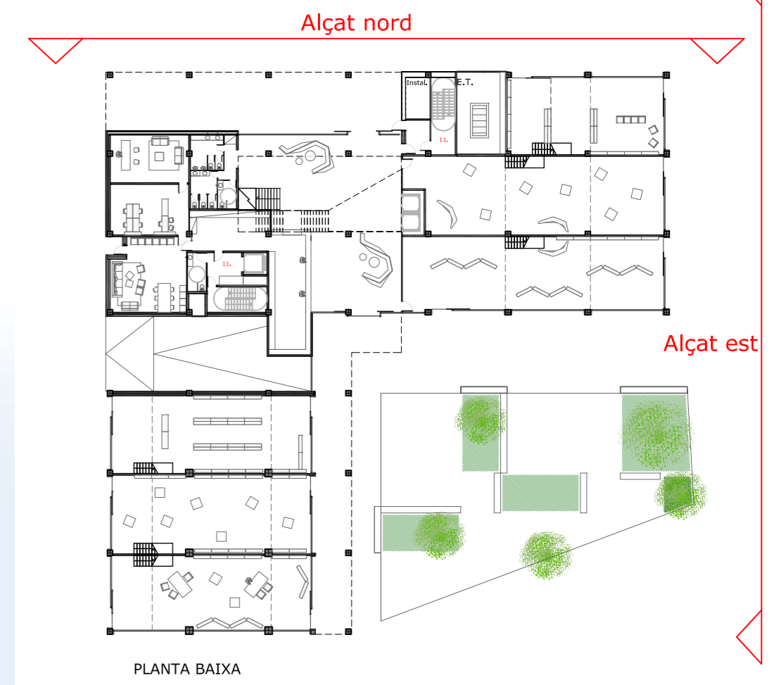
PLANTA BAIXA
