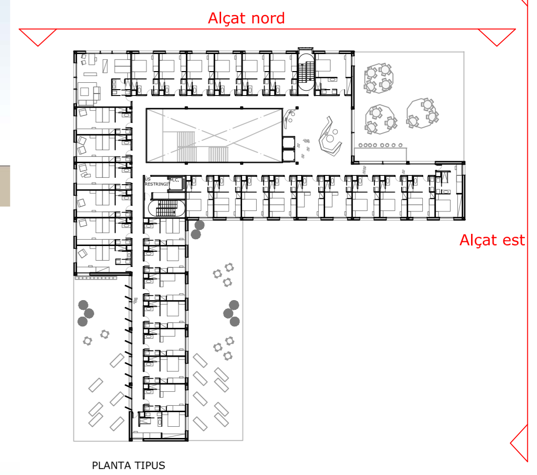
PLANTA TIPUS
