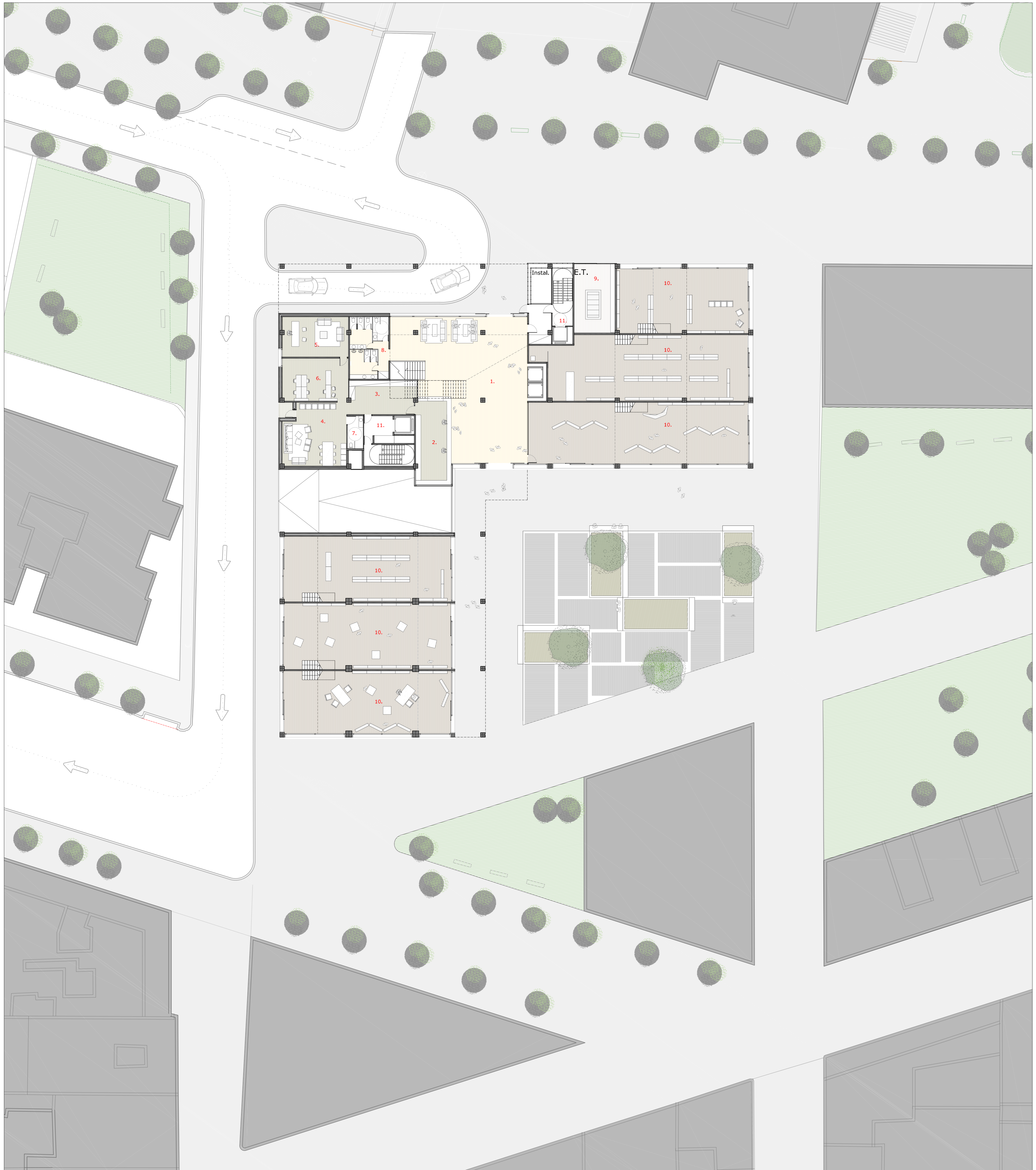
PLANTA BAIXA E:1/200
