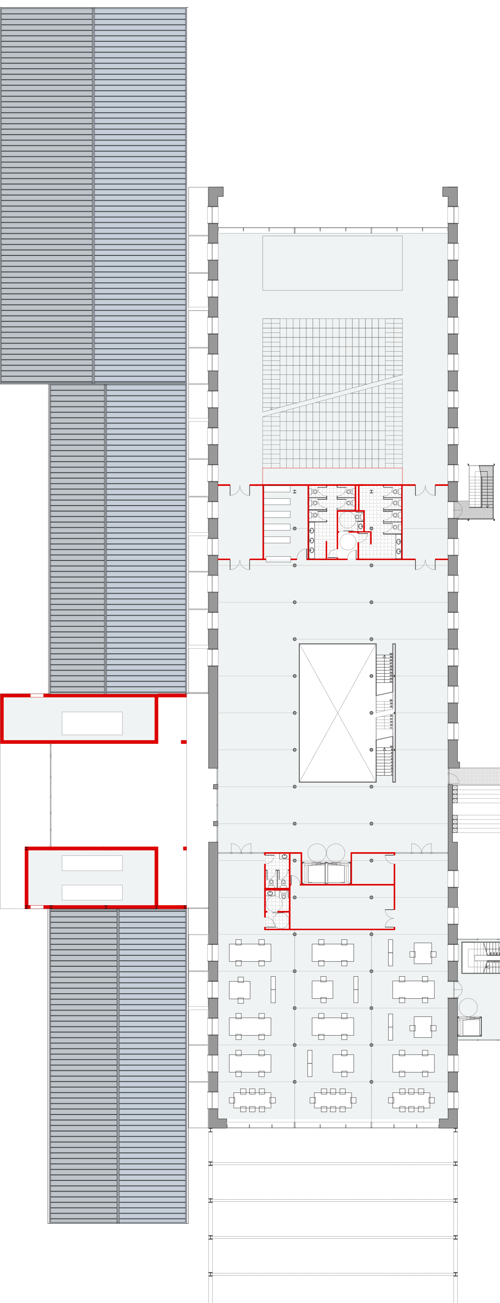
planta primera (cota +5,00m)
