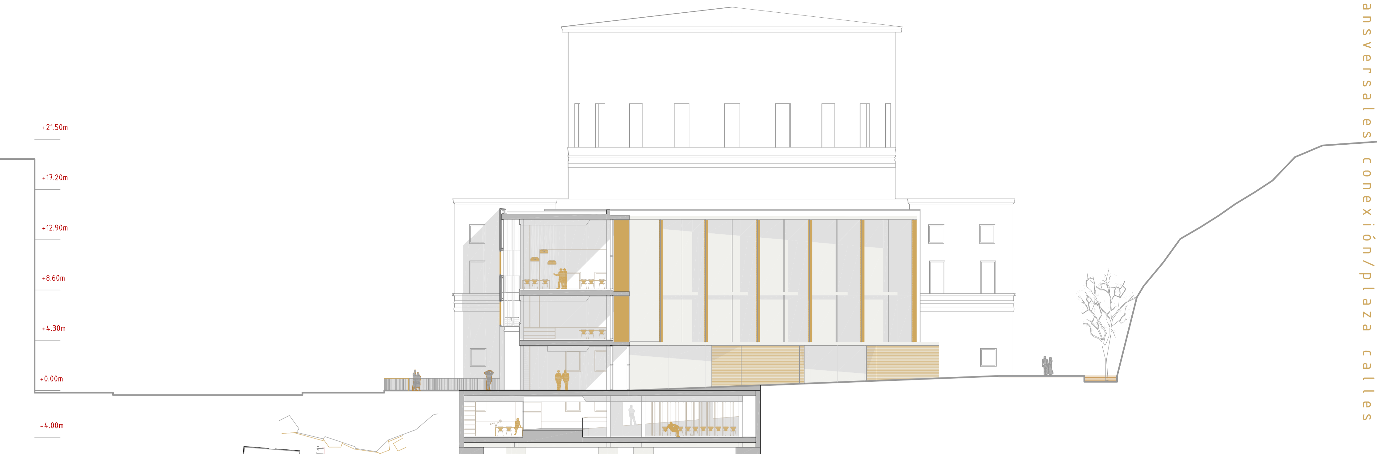
T1 sección transversal escala 1:200
