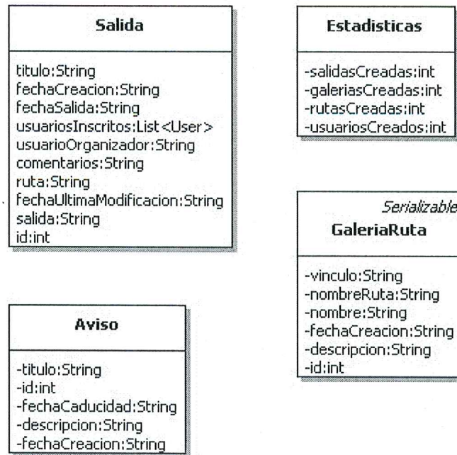
figura 21. Clases añadidas al modelo de la capa de servicios.
