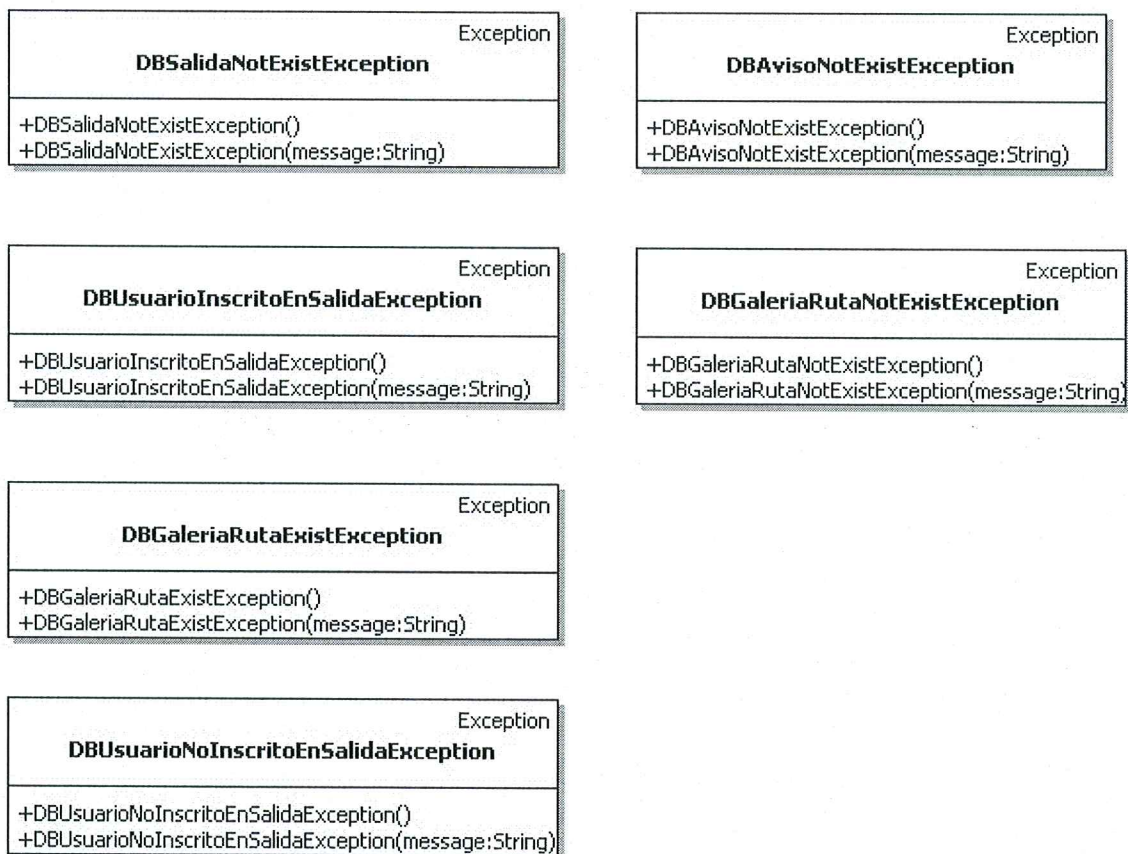
figura 22. Excepciones lanzadas por la capa de persistencia.
