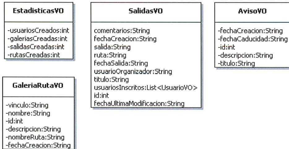
figura 25. Clases añadidas al modelo de la capa de persistencia.
