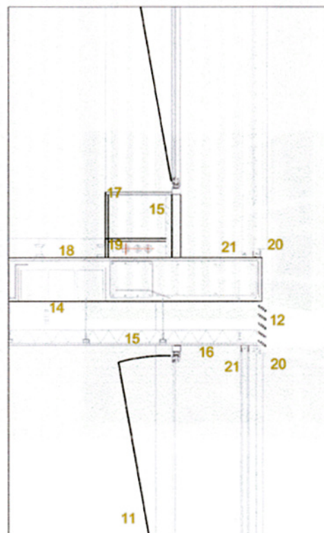
secció E: 1/20
