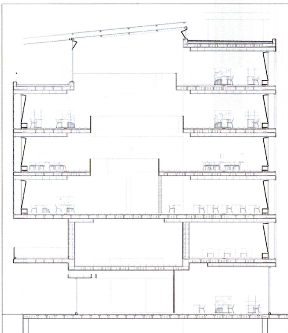
secció E: 1/50
