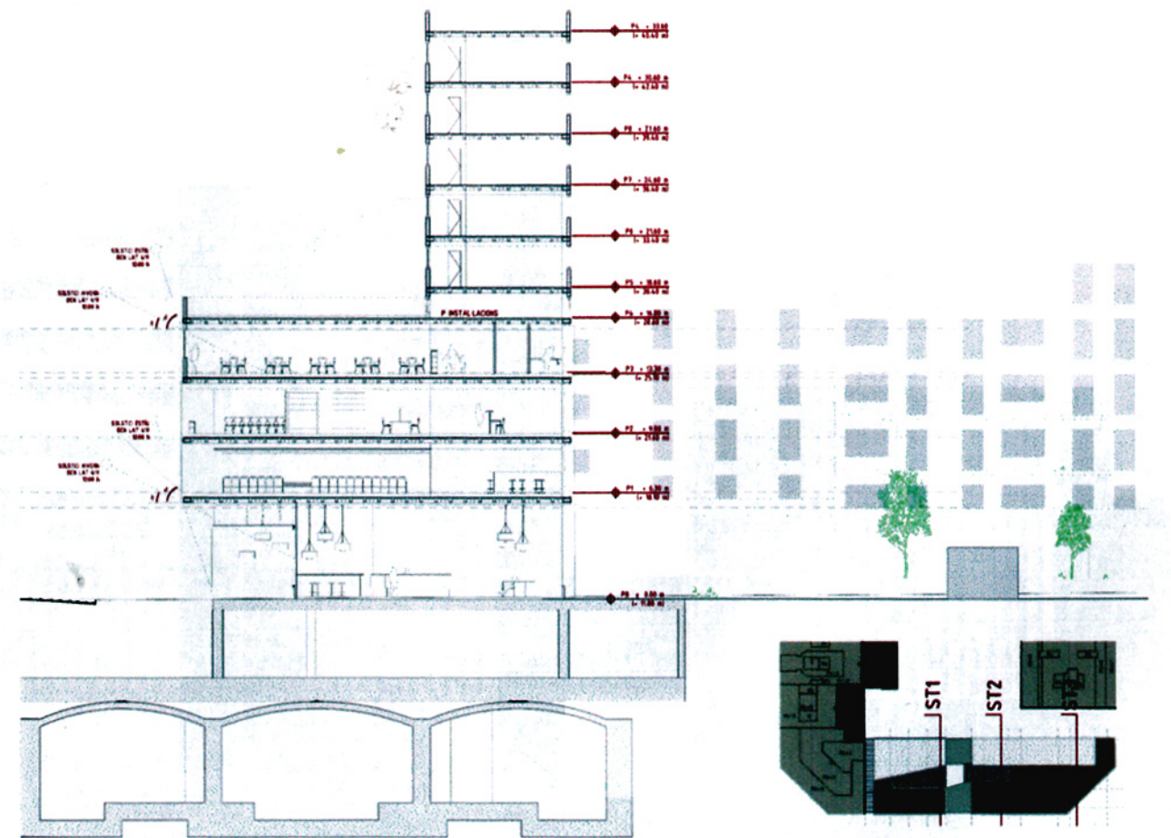
SECCIÓ TRANSVERSAL 3 e:1/200
