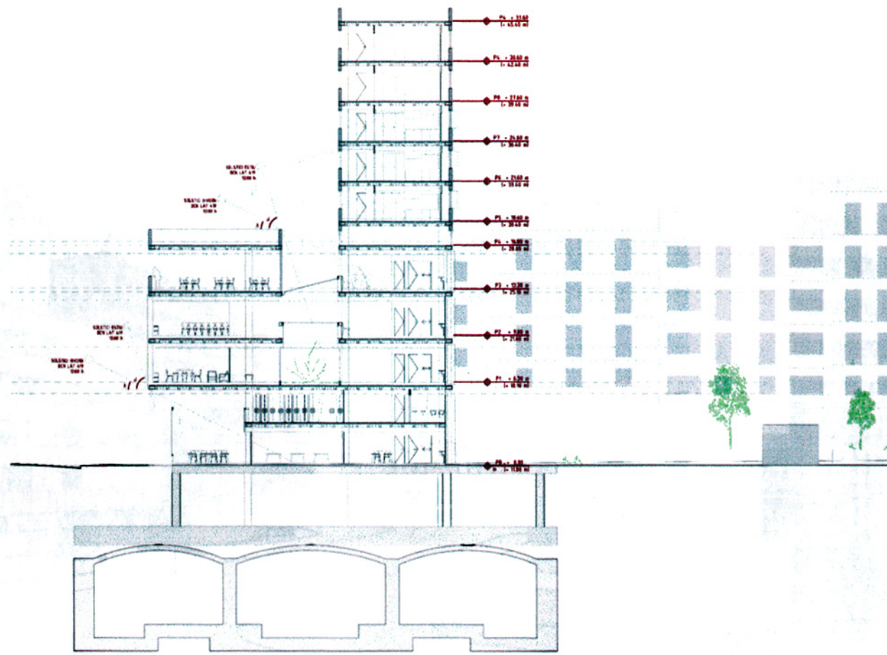
SECCIÓ TRANSVERSAL 2 e:1/200
