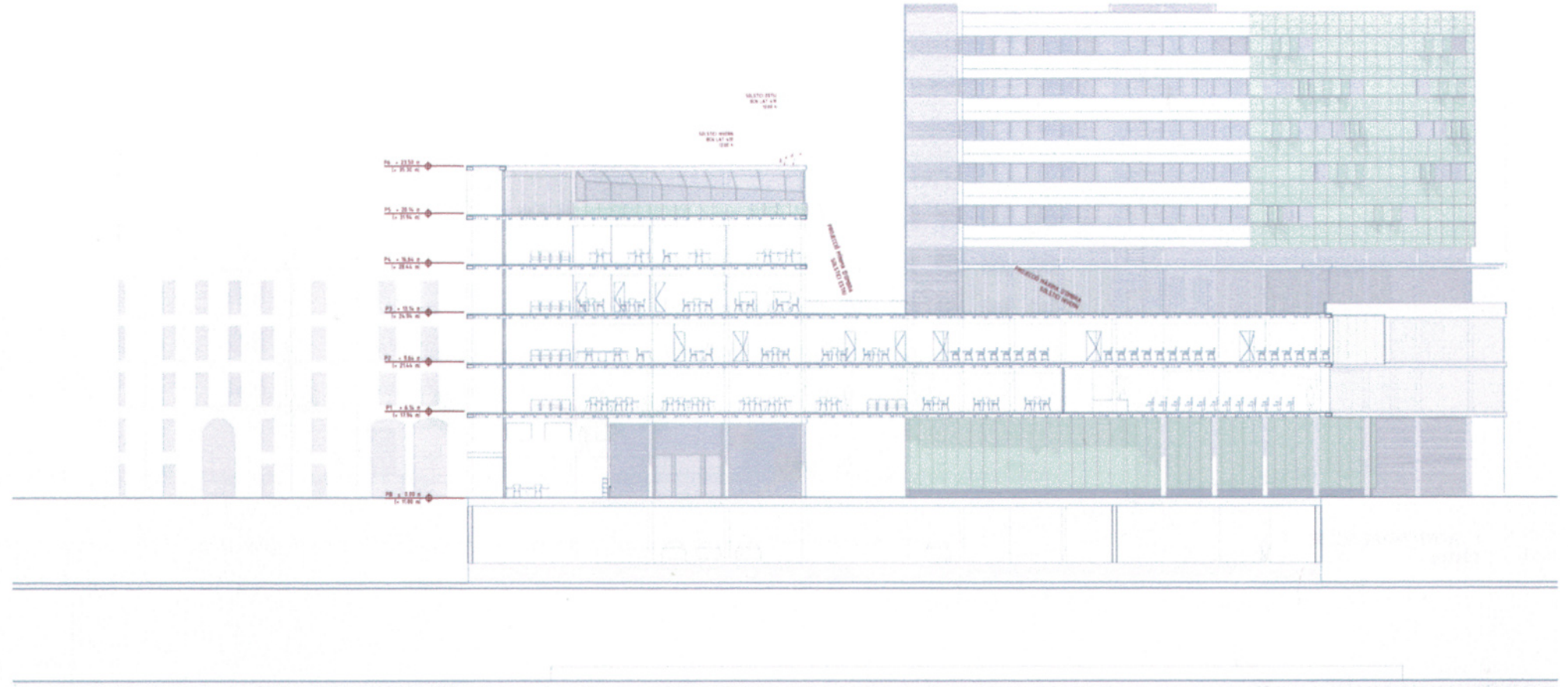
SECCIÓ LONGITUDINAL 1 e:1/200
