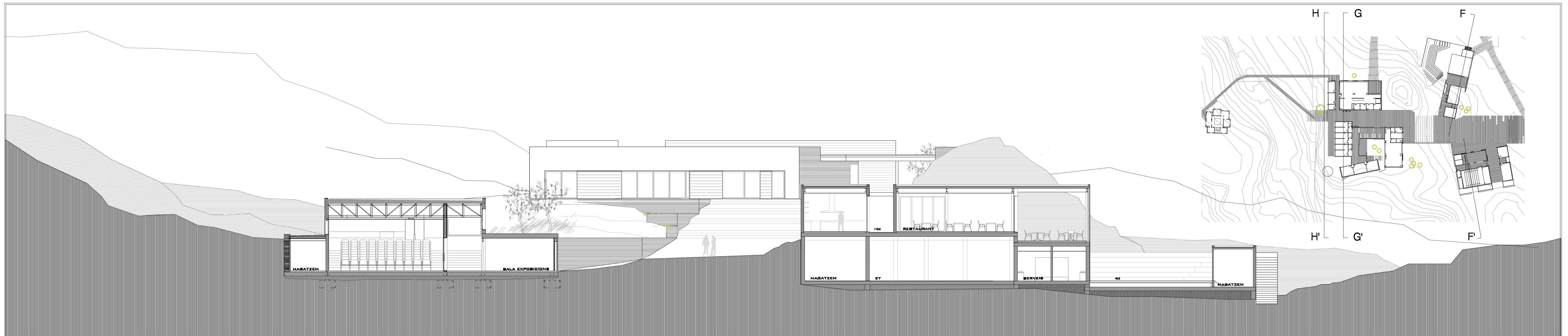
SECCIÓ F-F'
