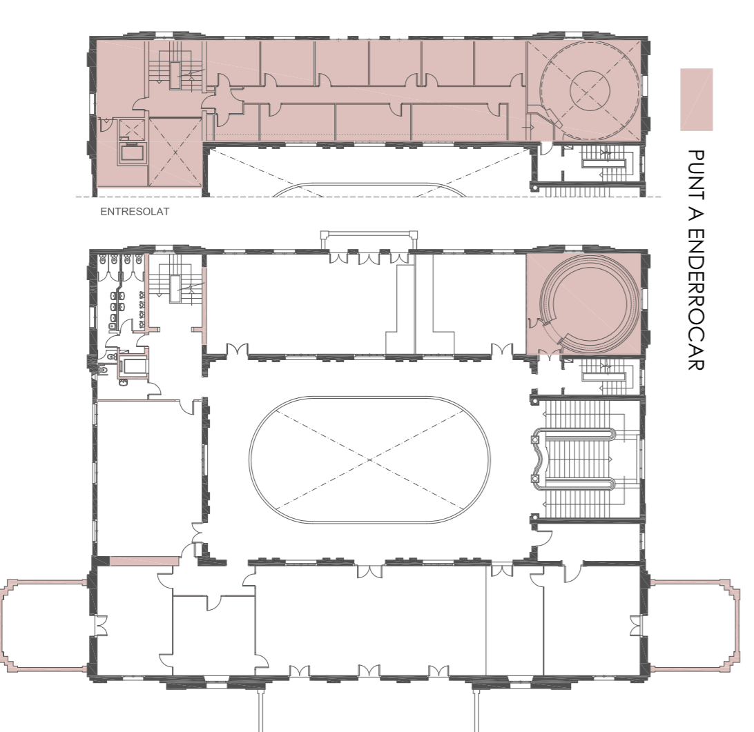
PLANTA PRIMERA - ENDERROCS
