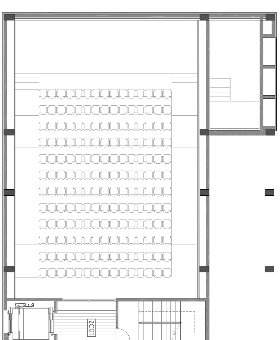
PLANTA ATELL AUDITORI
