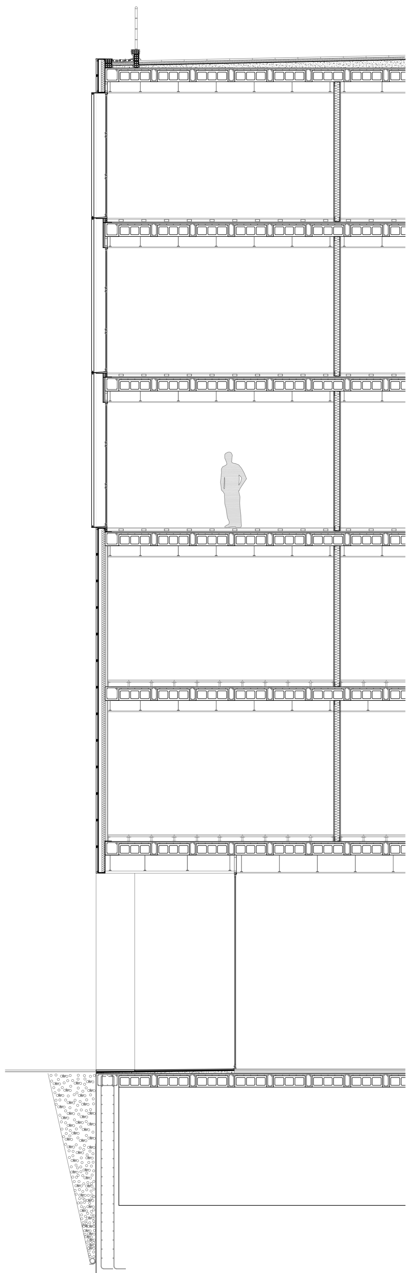
secció constructiva e:1/50
