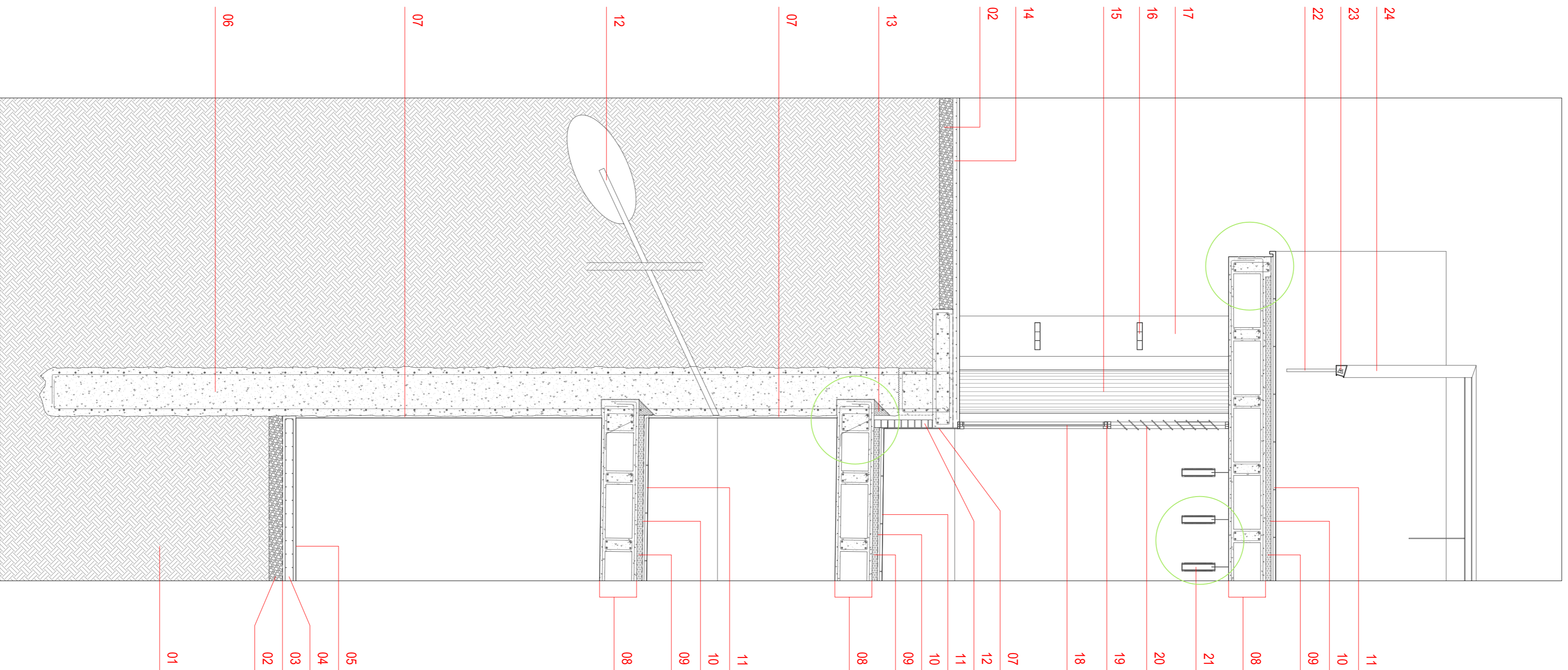
Secció tipus façana A1 e:1/50 A3 e:1/100
