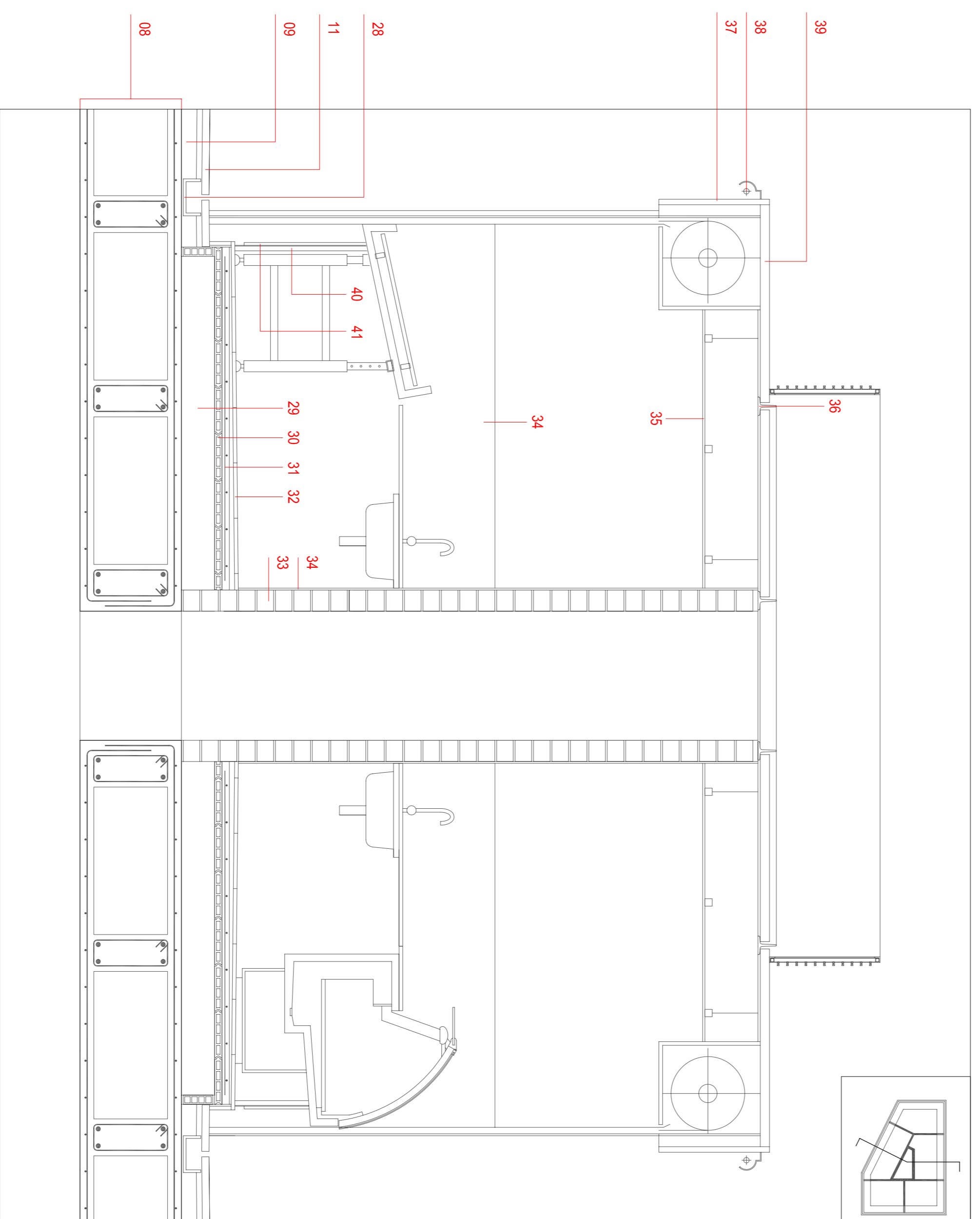
Secció tipus d'una illa de parades del mercat A1 e:1/20 A3 e:1/40
