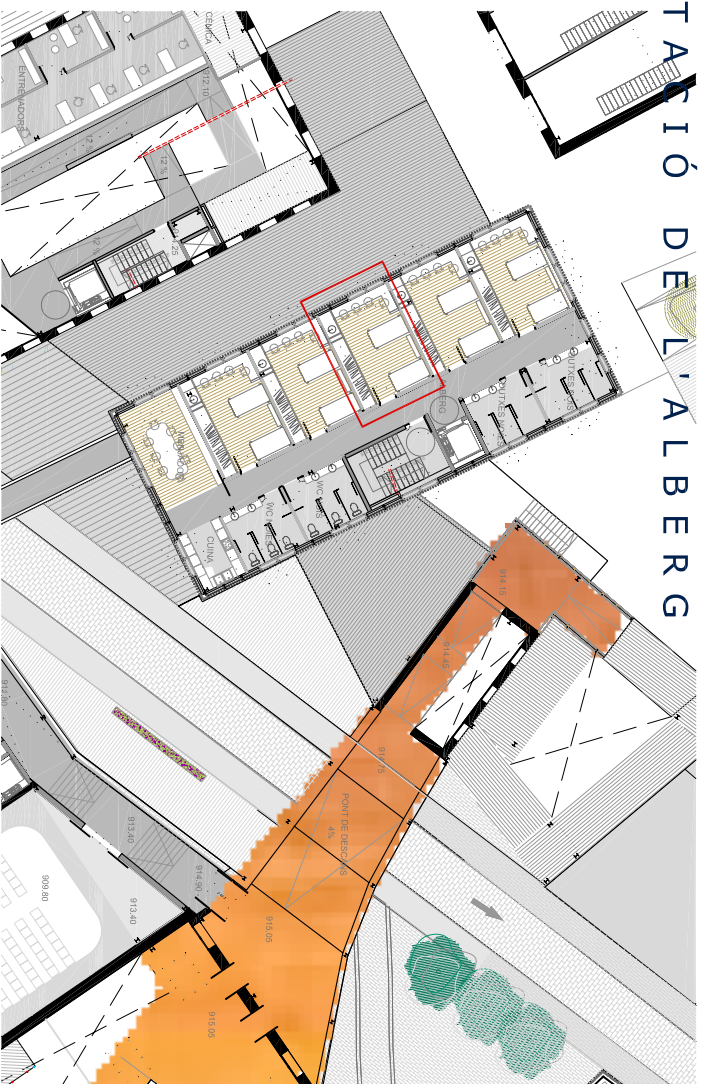
PLANTA DE L'ALBERG A1 E1:200 A3 E1:400
