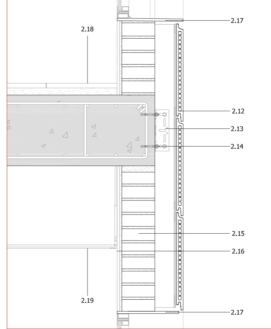
Detall plaques ceràmiques e 1/10
