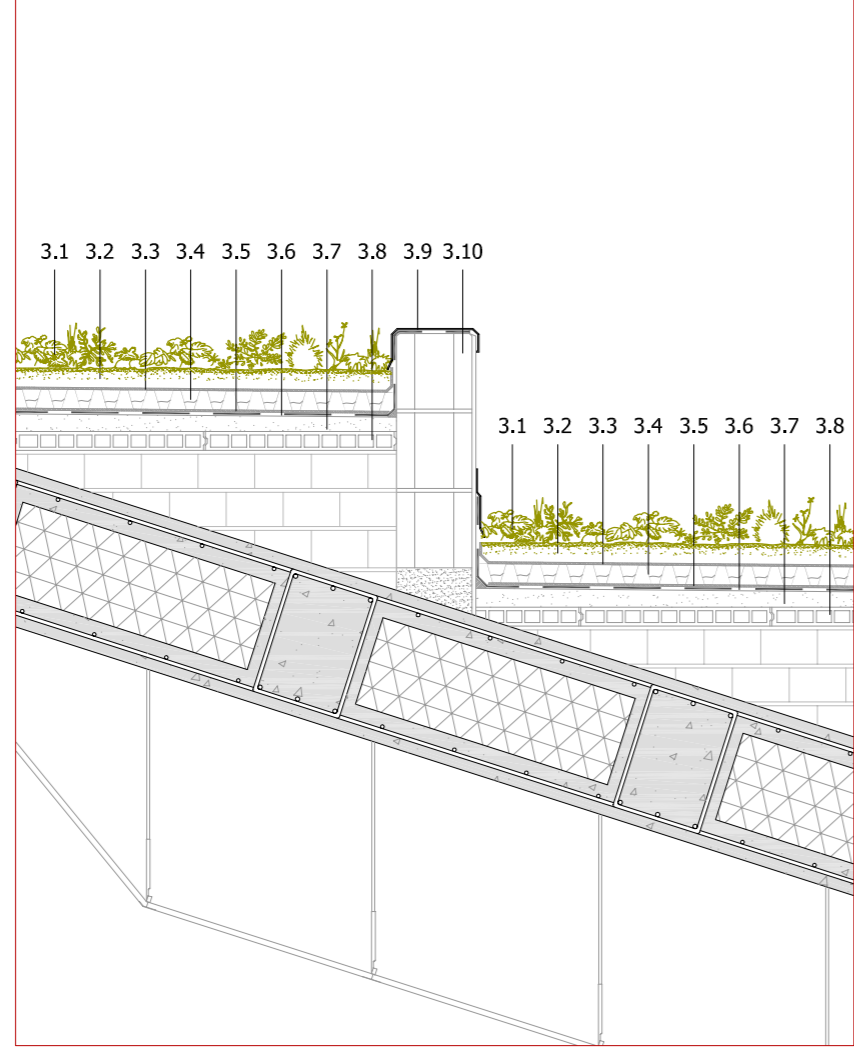
Secció 1 lames e 1/10
