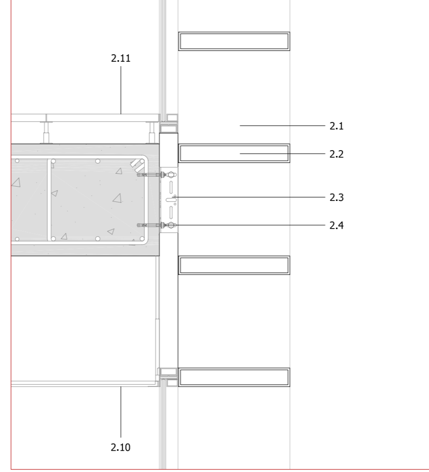
Detall proteccions alumini e 1/10
