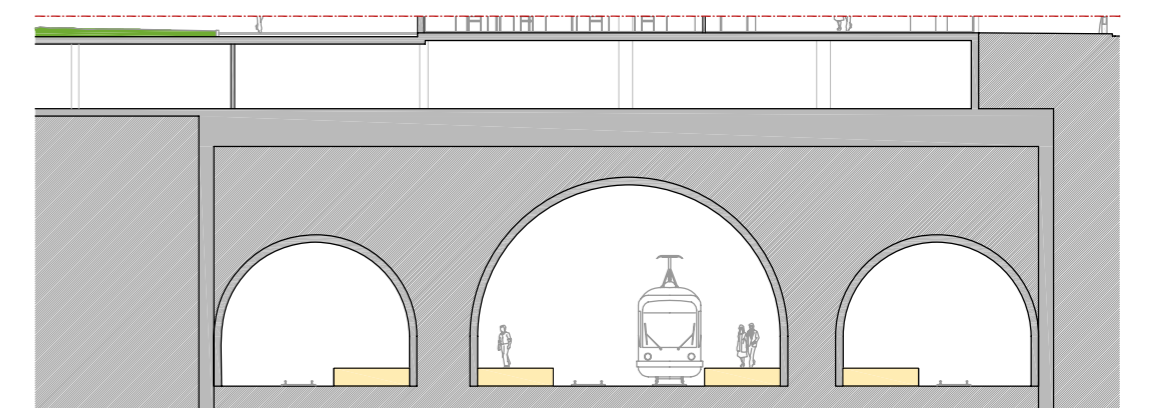
Secció tipus
