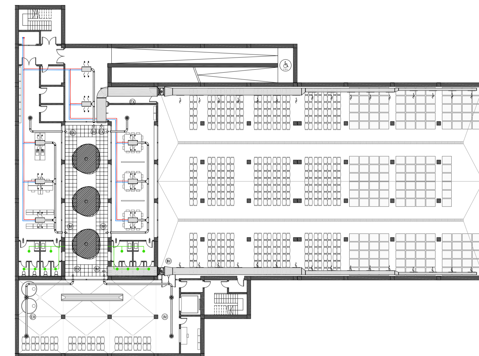
NIVELL 4 (COTA +288.00 m)
