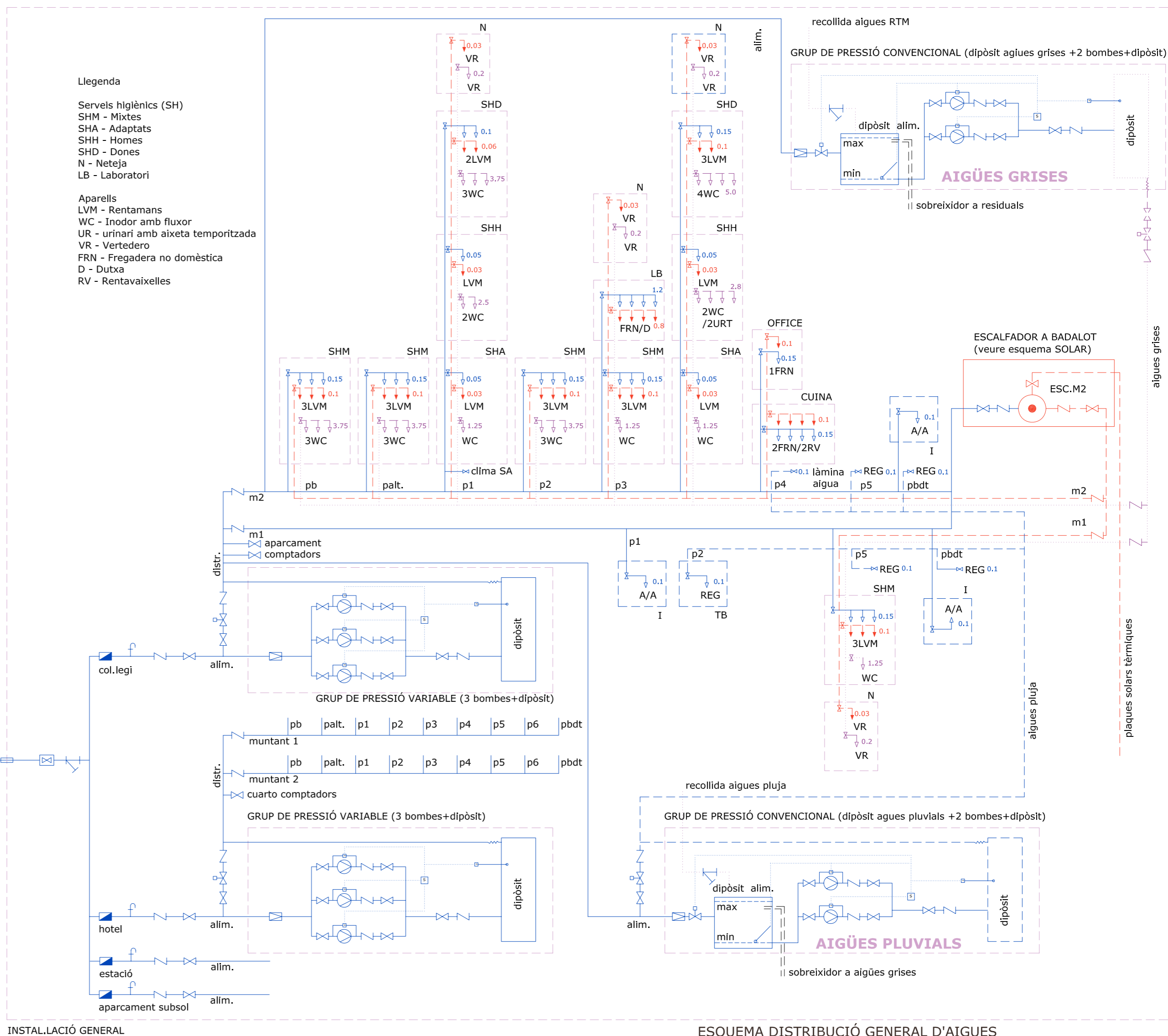
INSTAL·LACIÓ GENERAL
