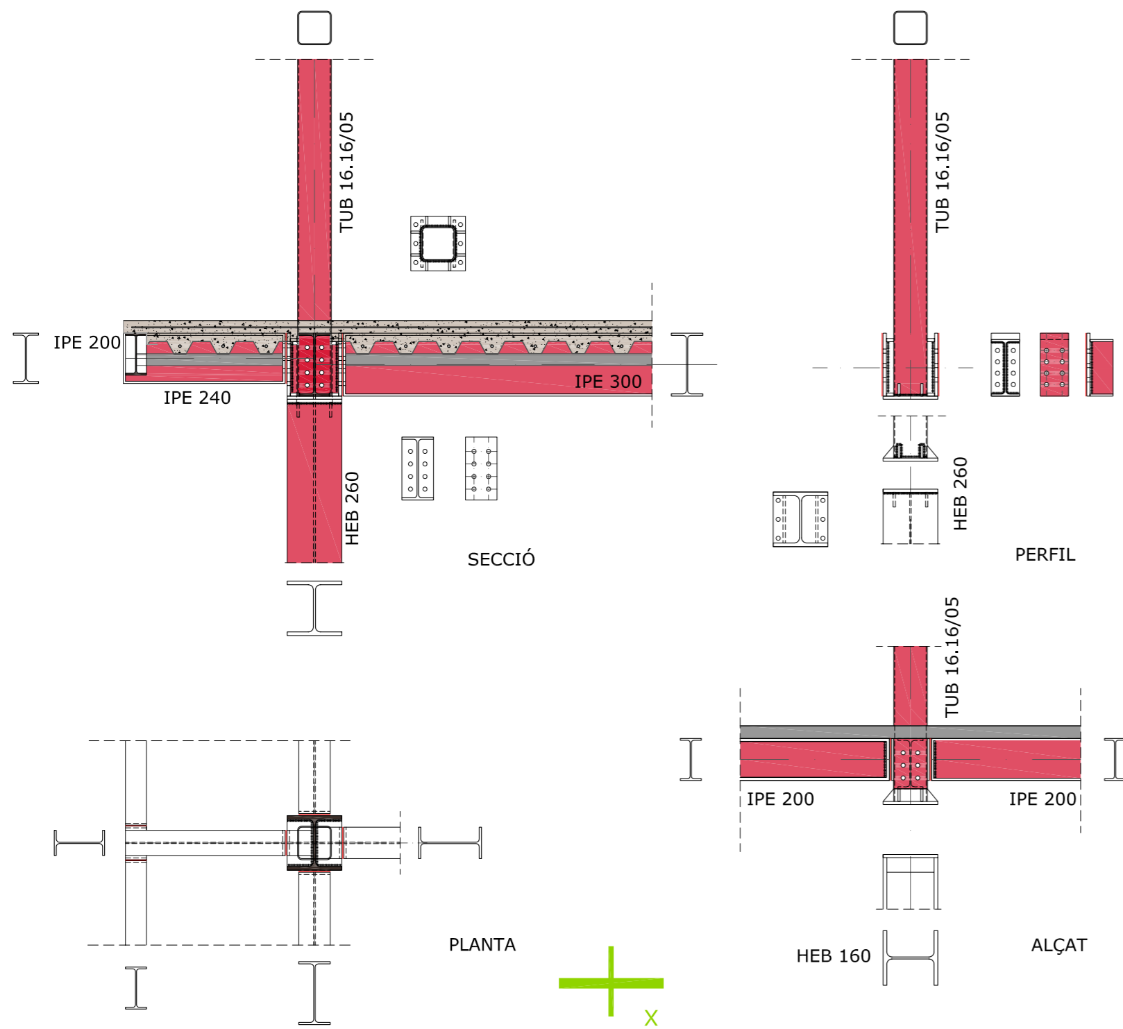
DETALL 7_UNIÓ RÍGIDA (X) AMB VOLADÍS_e:1/25
