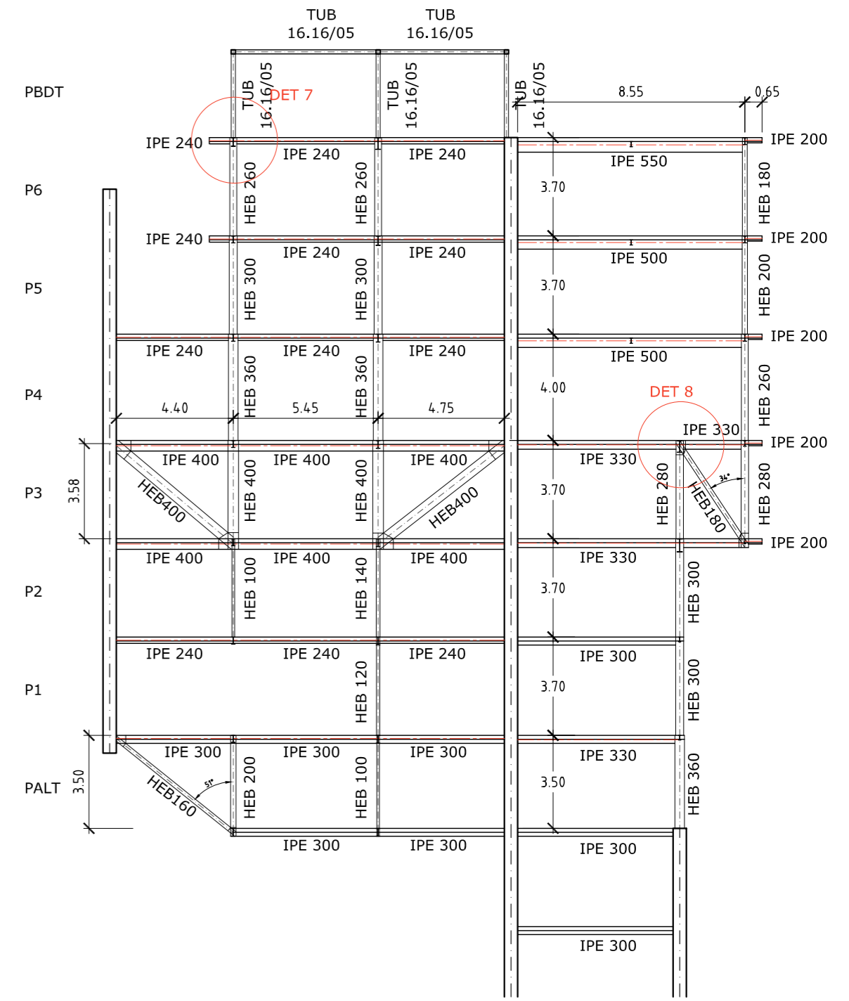
SECCIÓ PORTIC 4_e:1/200
