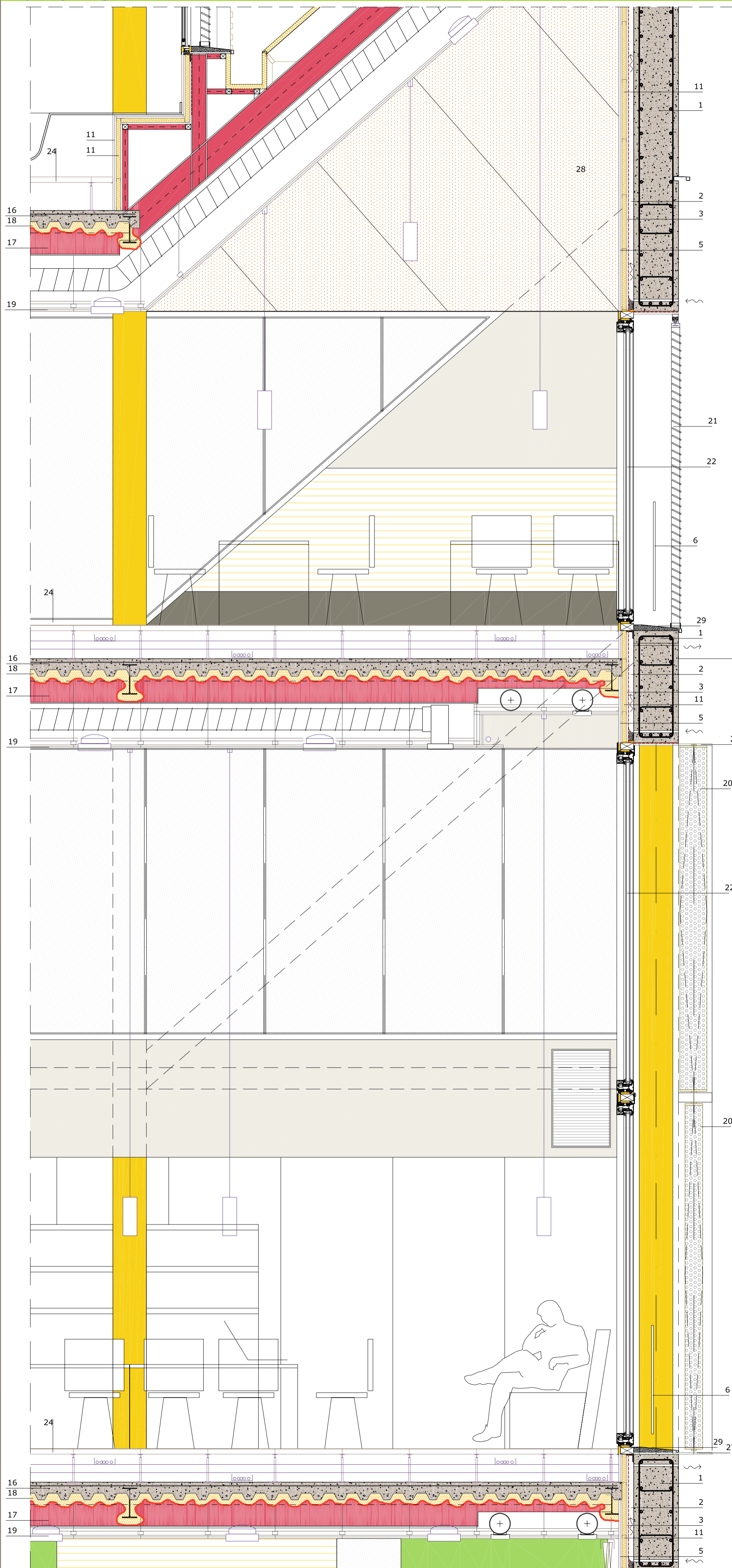
SECCIÓ CONSTRUCTIVA e/1:25
