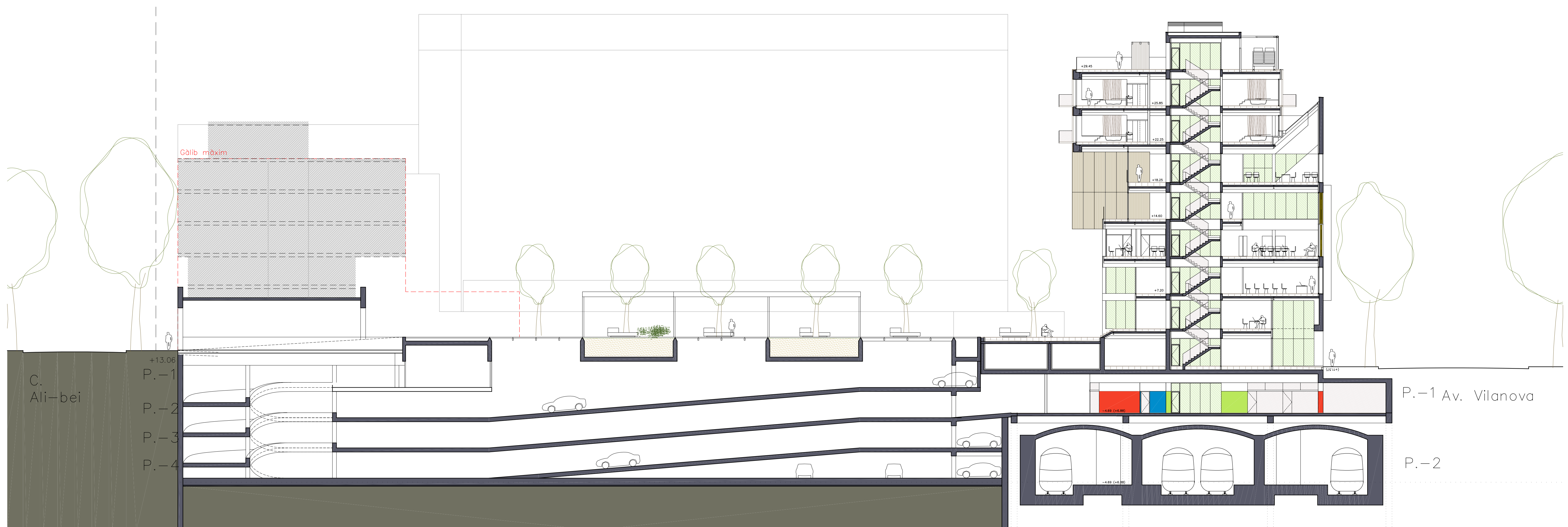
SECCIÓ T4 e/1:200
