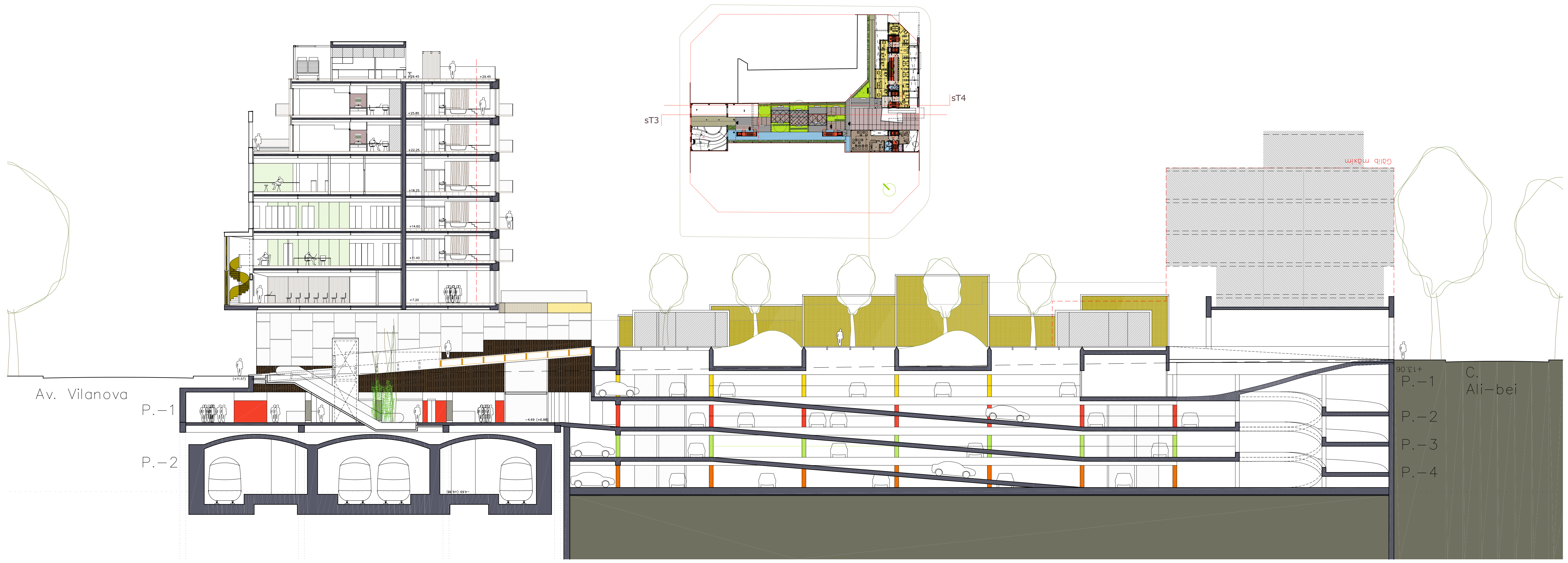
SECCIÓ T3 e/1:200
