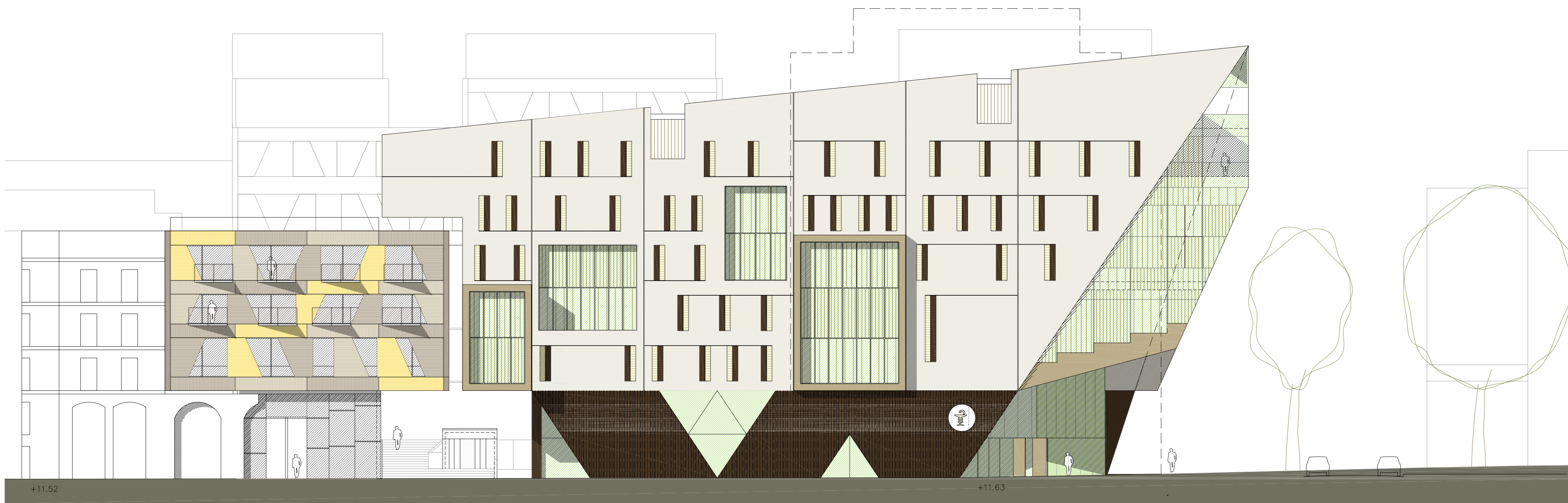
FAÇANA AV. VILANOVA e/1:200
