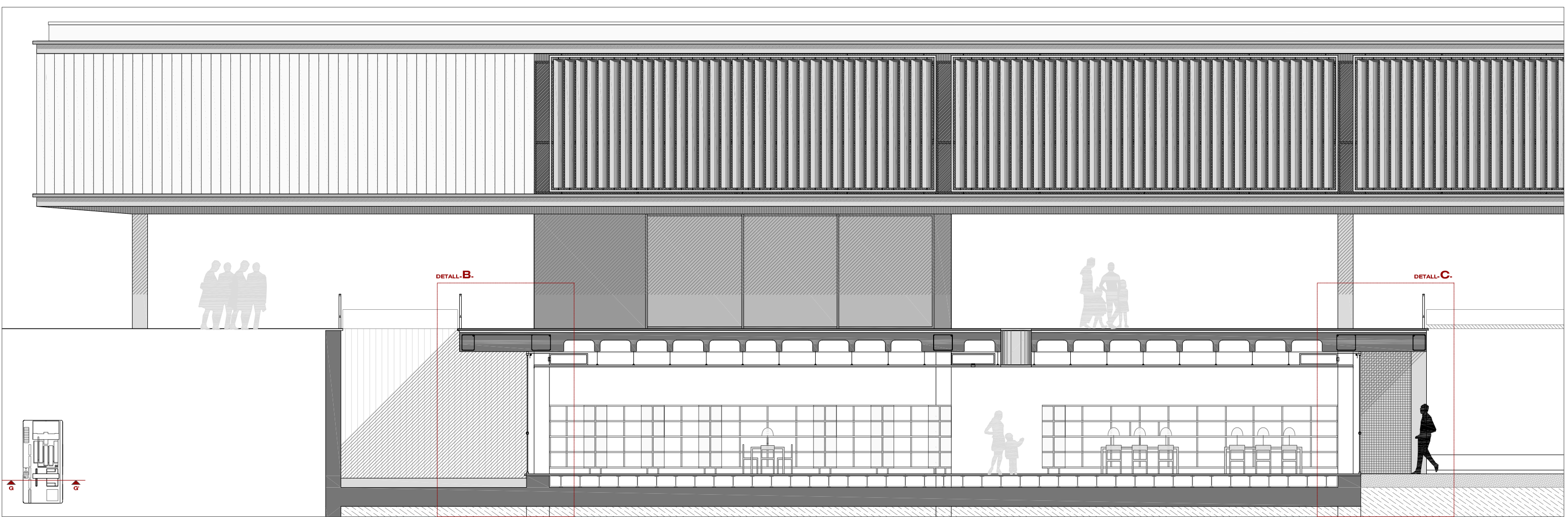
-SECCIO OEST G-G-
