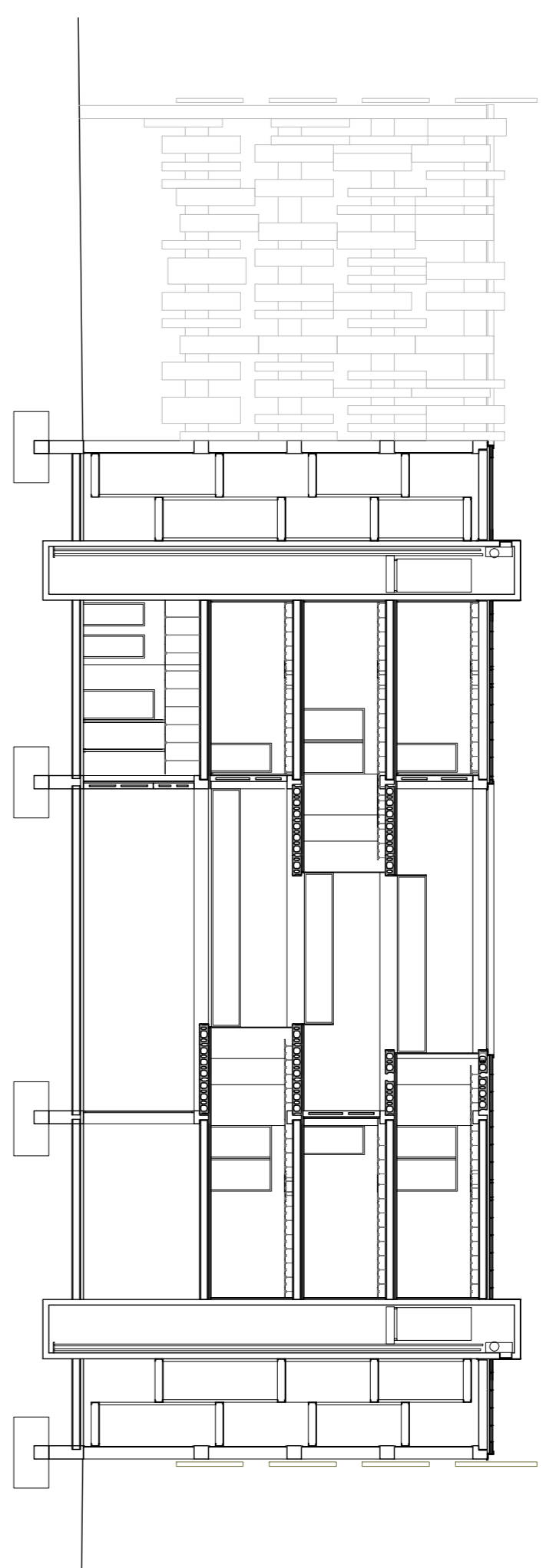
Secció 1-1
