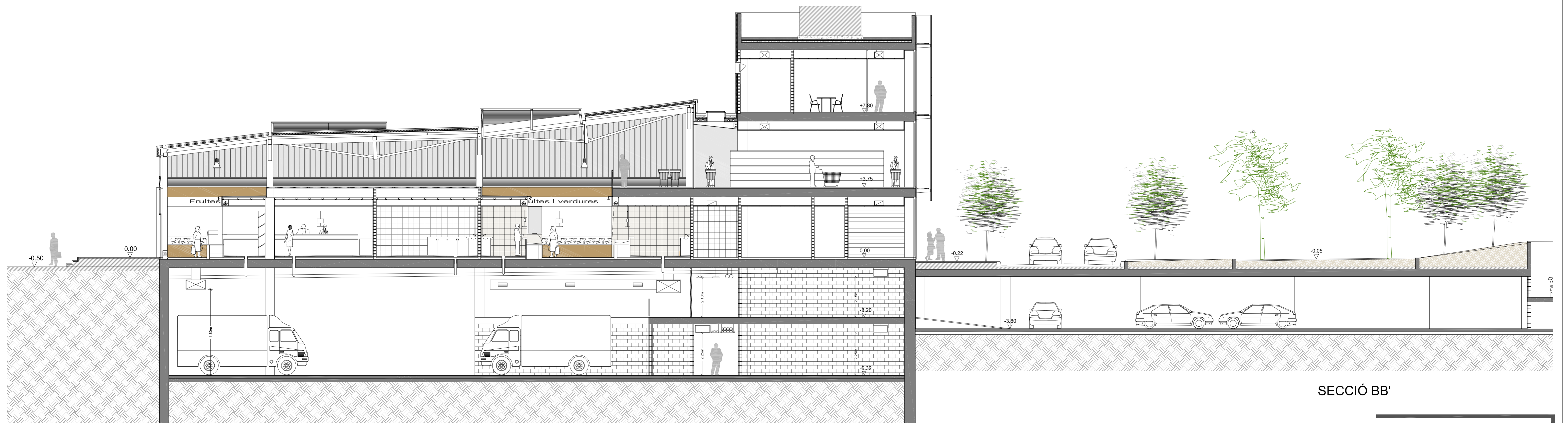
SECCIÓ AA'
