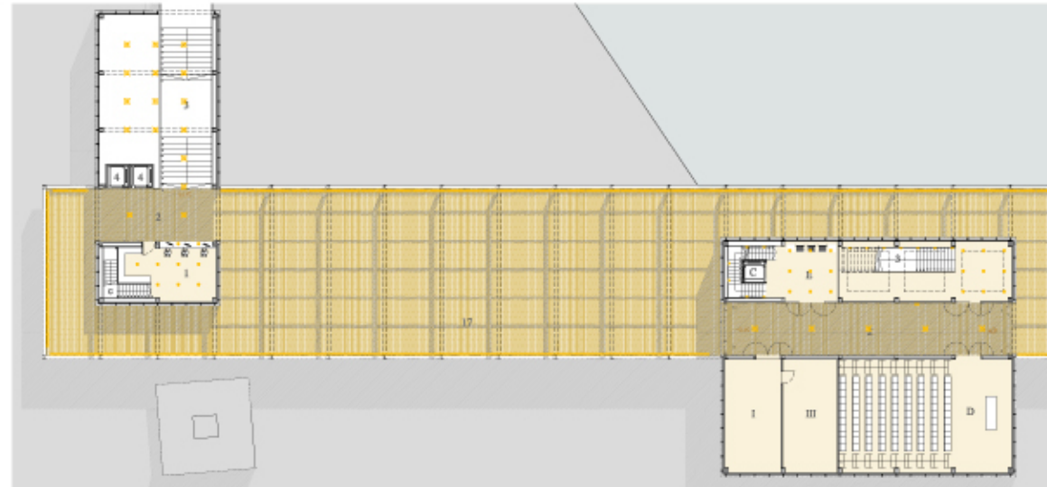
TAQUILLES/AUDITORI PLANTA PRIMERA E: 1/300
